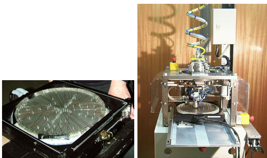
FIGURE 2.2 – A gauche : vue d'une plaque de fibres prête à être montée dans le plan focal du télescope. A droite : vue du robot positionneur de fibre. Lors d'une observation, pendant que l'intégration sur le ciel est en cours, le robot prépare la plaque suivante. Le projet RAVE dispose de 3 plaques pour palier aux temps morts dus à la réparation de fibres sur ces dernières.
