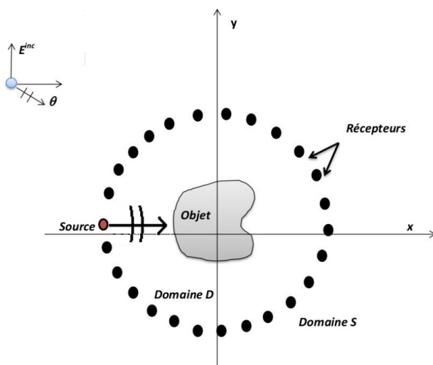
FIGURE 2.1 – La configuration en imagerie micro-onde bi-dimensionnelle en polarisation transverse magnétique (2D-TM).
