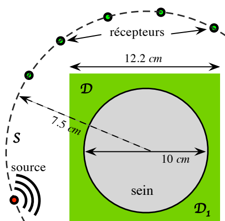
FIGURE 2.3 – Configuration de mesure
