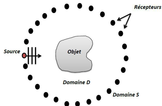
FIGURE 1.3 – Configuration géométrique en imagerie micro-onde bi-dimensionnelle (2D)
