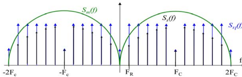
Figure 35: Galileo E1OS code spectrum
