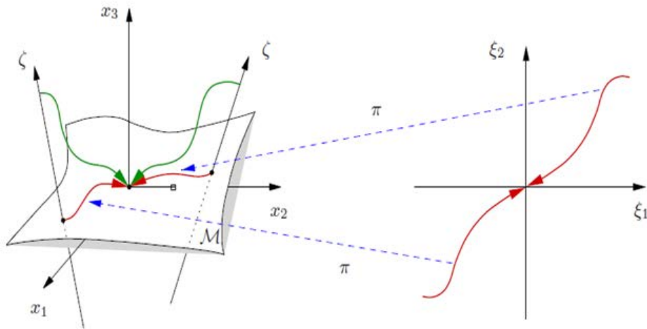
Figure 5.1 : Principe de la commande I&I [Astolfi et al., 2008]
