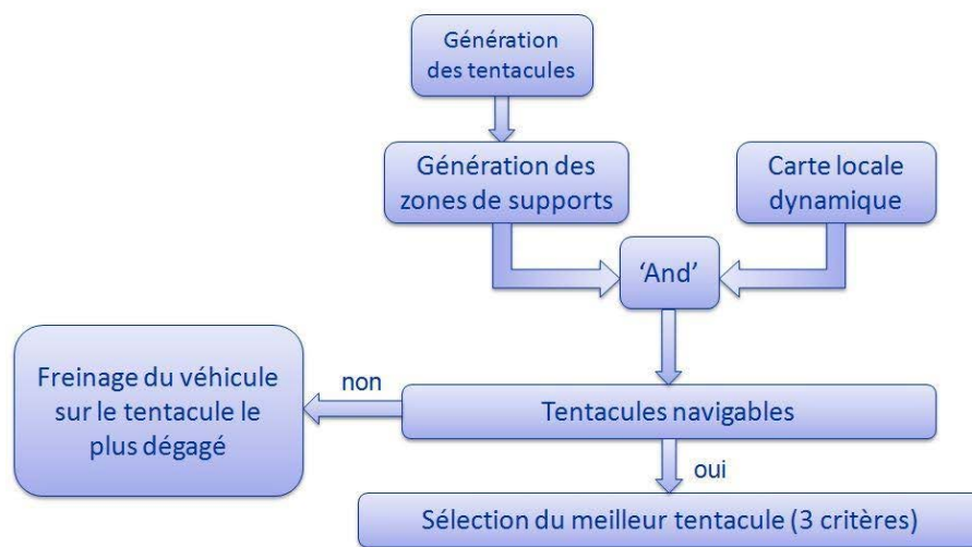
Figure 8.7 : Algorithme de navigation par la méthode des tentacules [Tang et al., 2013]
