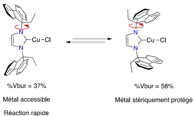
Schéma 10 : Encombrement stérique variable dans le complexe [\text{CuCl}(\text{imidazolylidène } \text{E}_f/\text{EF})] .
