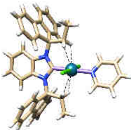
Figure 1 : Structure cristallographique d'un complexe Pd-PEPPSI-NHC obtenu à partir d'un NHC substitués par deux groupes AF (ici 9-éthyl-9-fluorényle).
