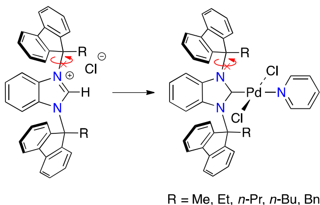
Schéma 2 : Synthèse des complexes (Pd-PEPPSI-NHC).
