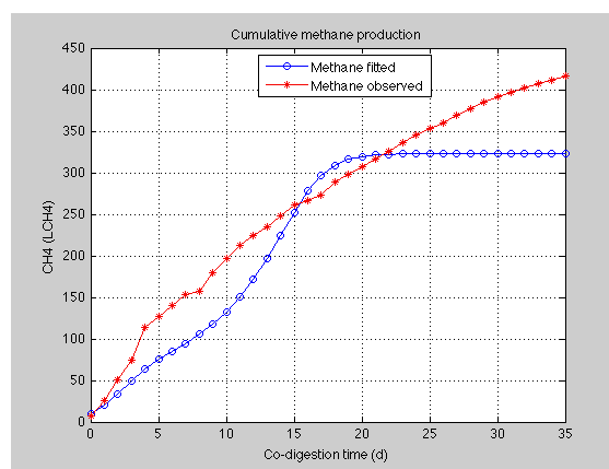
Figure V-18 : Production cumulée de méthane mesurée expérimentalement (mélange n°4) et simulée par le modèle de Couplage
