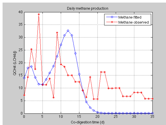
Figure V-13 : Production journalière de méthane mesurée expérimentalement (mélange n°5) et simulée par le modèle de Couplage
