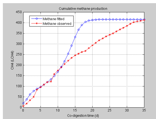
Figure V-16 : Production cumulée de méthane mesurée expérimentalement (mélange n°8) et simulée par le modèle de Couplage
