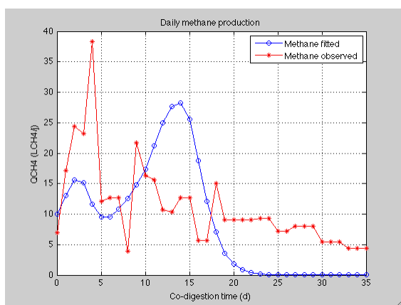
Figure V-17 : Production journalière de méthane mesurée expérimentalement (mélange n°4) et simulée par le modèle de Couplage
