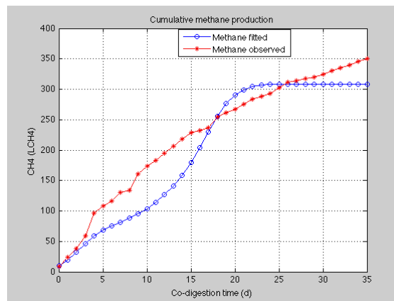
Figure V-20 : Production cumulée de méthane mesurée expérimentalement (mélange n°9) et simulée par le modèle de Couplage
