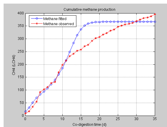
Figure V-8 : Production cumulée de méthane mesurée expérimentalement (mélange n°1) et simulée par le modèle de Couplage
