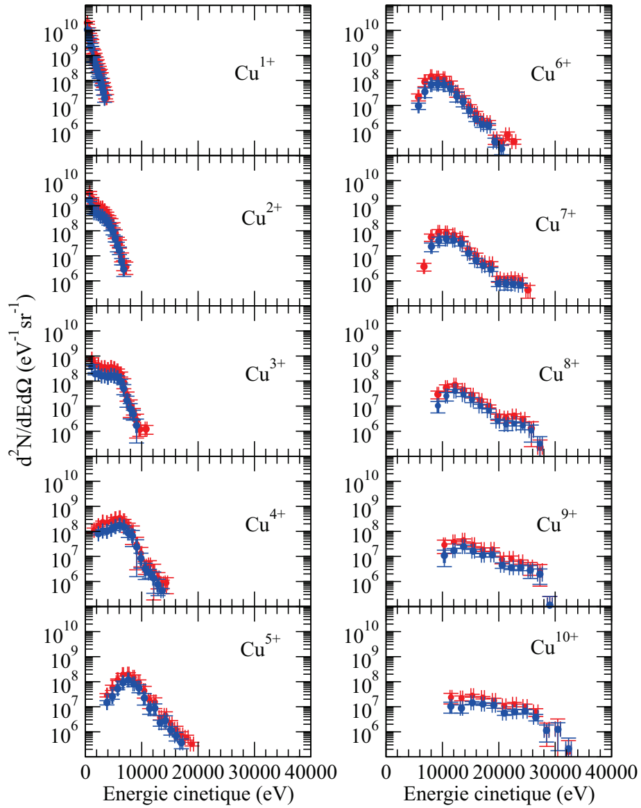
FIGURE 4.32 – Distribution en énergie "équivalente" des ions cuivre, d'états de charge 1^+ à 10^+ à l'entrée du déviateur qui est considéré comme idéal. La courbe rouge représente les ions de ^{63}\text{Cu} et la courbe bleue ceux du ^{65}\text{Cu}
