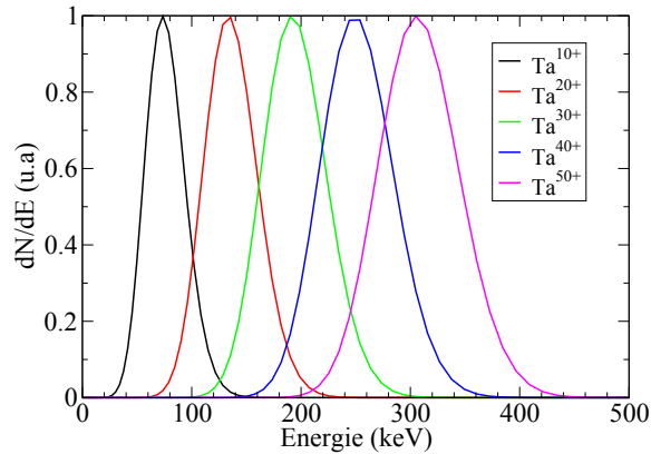
FIGURE 4.48 – Distribution en énergie des ions tantales à 10^{14} W/cm 2 pour des états de charge de 10^+ à 50^+ .
