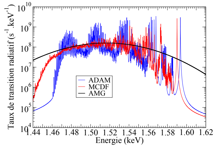
FIGURE 2.25 – Comparaison des trois approches sur la transition 6p_{1/2}-4p_{3/2} pour une température de plasma de 316 eV et une densité de 10^{-2} g/cm ^3 . Les états de charge calculés avec ADAM et MCDF vont de 47^+ à 51^+ .
