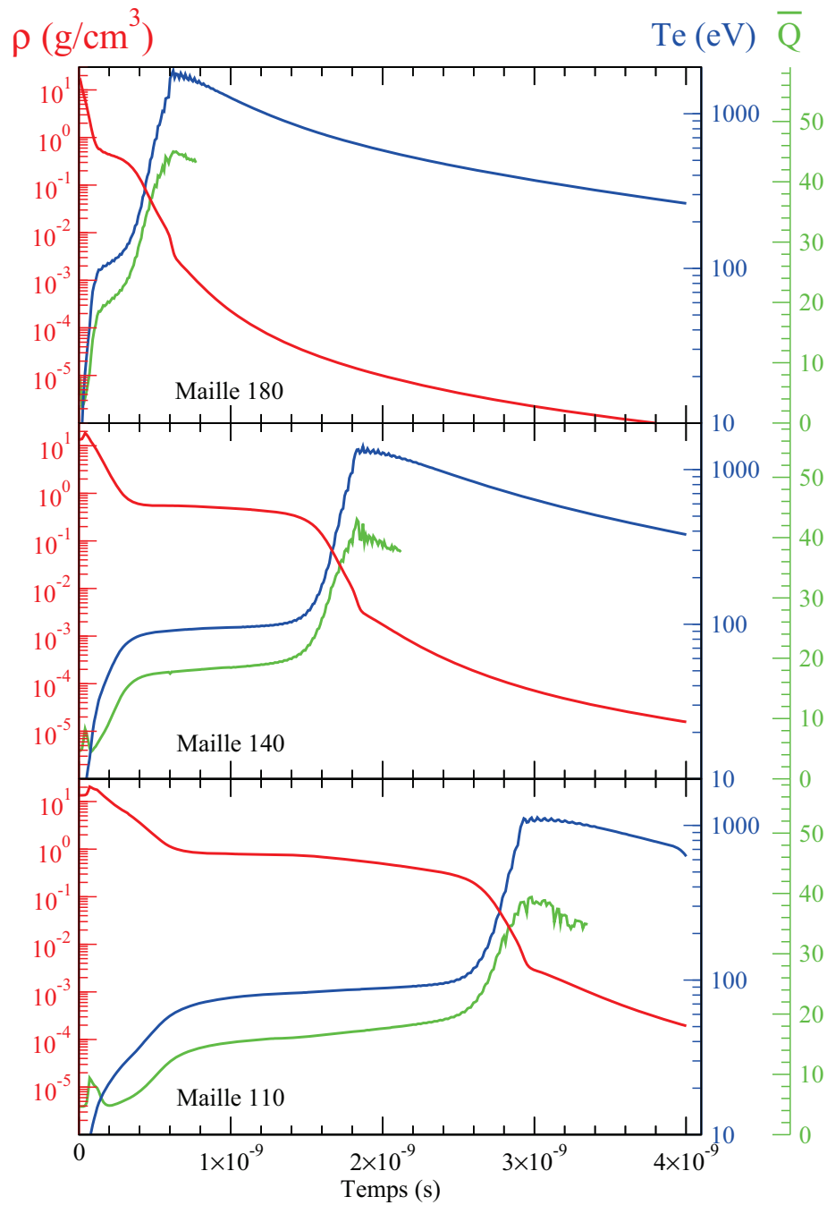
FIGURE 3.8 – Variation de la densité (en rouge), de la température en eV (en bleu) et de l'état de charge moyen (en vert) en fonction du temps pour les mailles 180, 140 et 110. L'état de charge est calculé en postprocesseur par NOHEL2e pour des densités supérieures à 10^{-3} g/cm 3 .
