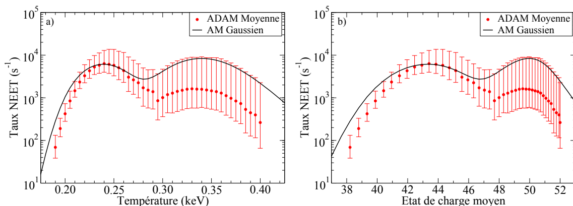
FIGURE 2.32 – Évolution de la moyenne taux NEET pour un plasma de ^{201}\text{Hg} à 10^{-2} \text{g}/\text{cm}^3 et de sa dispersion en fonction a) de la température et b) de l'état de charge moyen.
