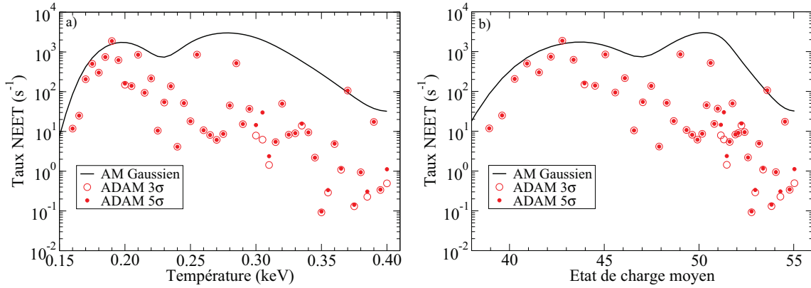
FIGURE 2.29 – Comparaison des taux NEET calculés avec l'AMG et ADAM à 10^{-3} g/cm 3 en fonction a) de la température et b) de l'état de charge moyen.
