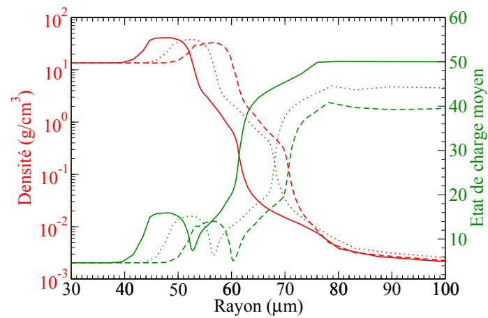
FIGURE 3.13 – Profil de densité (en rouge) et état de charge moyen (en vert) en fonction du rayon pour 3 intensités laser : 2 \times 10^{14} W/cm 2 (tirets), 5 \times 10^{14} W/cm 2 (pointillés) et 10^{15} W/cm 2 (trait plein).
