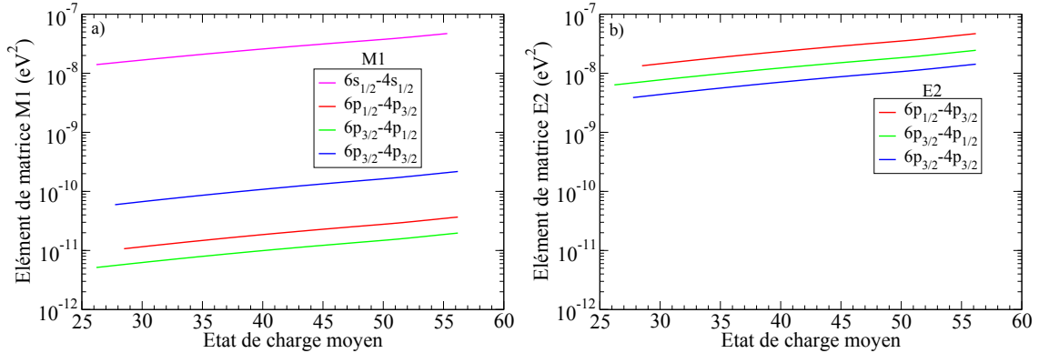
FIGURE 2.6 – Variation de l'élément de matrice de couplage en fonction de l'état de charge moyen pour a) la composante M1 et b) la composante E2.
