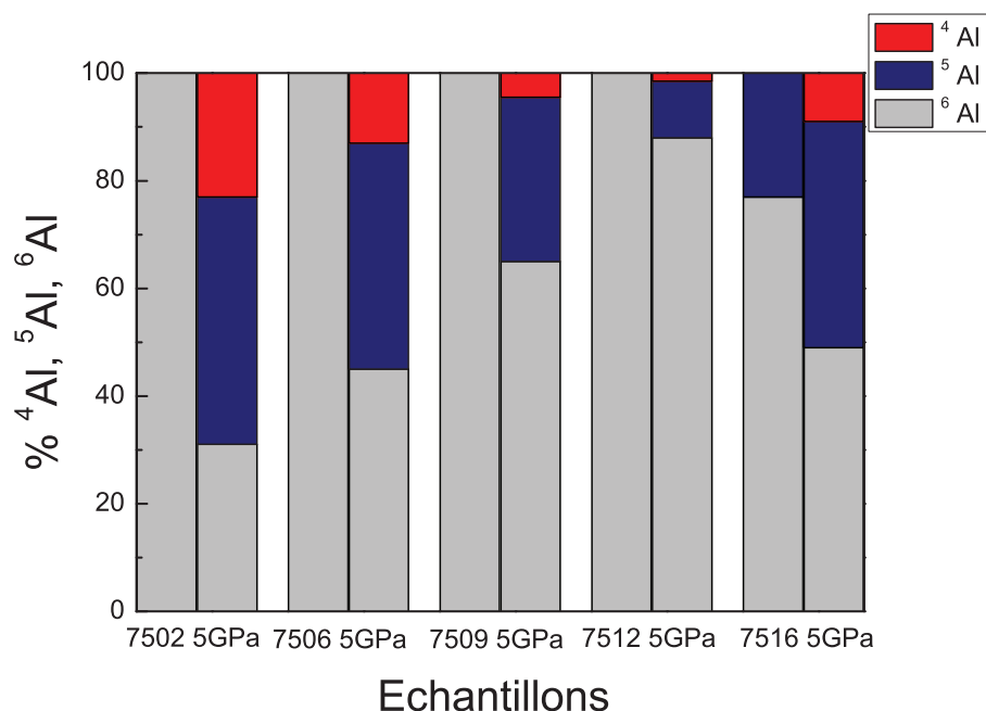
FIGURE 6.9 – Évolution des proportions d' 4 Al, d' 5 Al et d' 6 Al déterminées grâce au programme dmfit. Les résultats sont regroupés deux par deux par composition en Al 2 O 3 avant (à gauche) et après densification (à droite) pour les échantillons 7502, 7506, 7509, 7512 et 7516.
