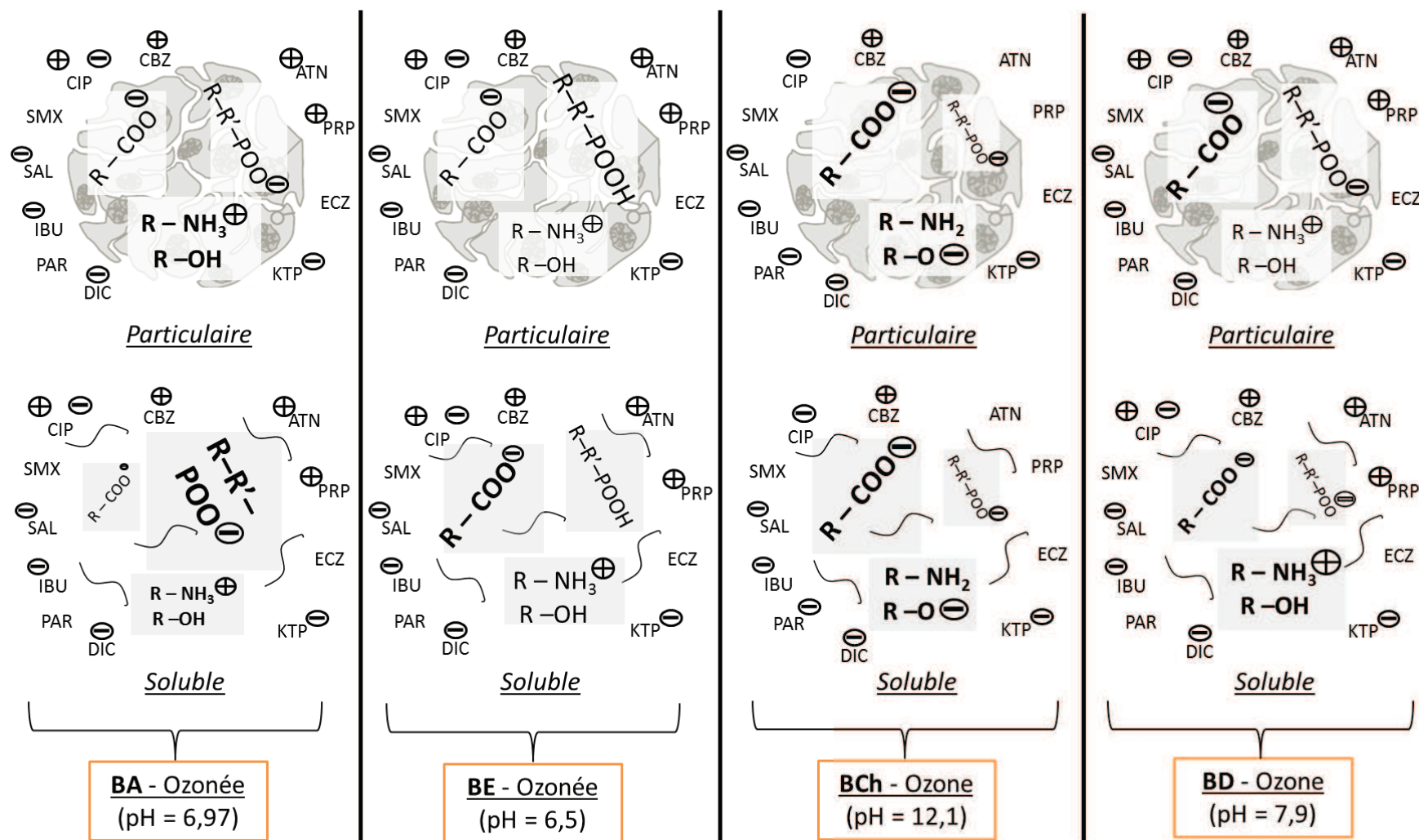
Figure 58 : Schématisation de la répartition des charges et des groupements fonctionnels pour les interactions boues/micropolluants au cours du traitement (lot des boues urbaines ozonées)
