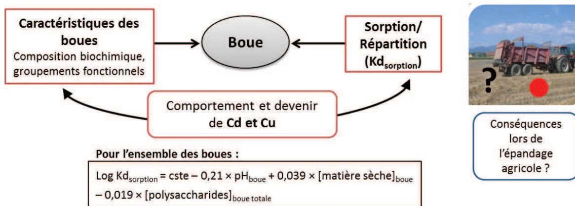
Figure 99 : Modélisation de K_{d_{sorption}} pour les métaux Cd et Cu
