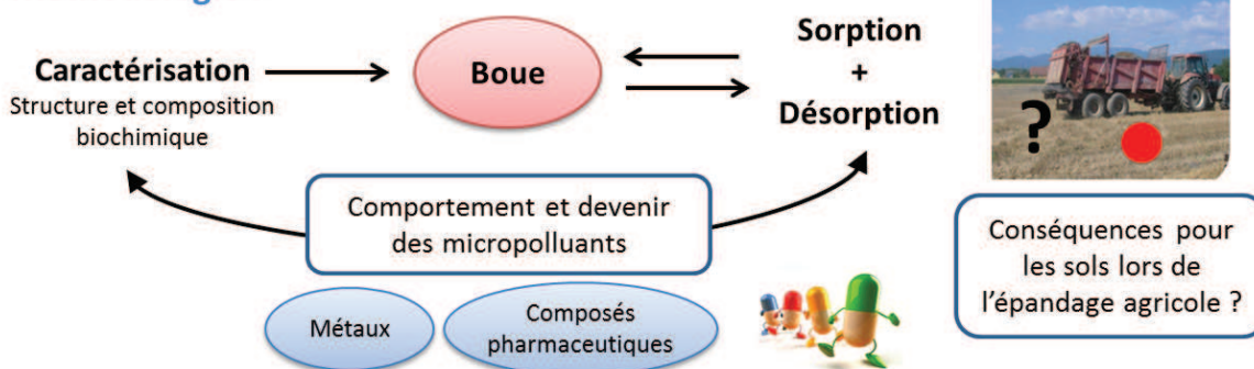
Figure 33 : Schématisation de la problématique et de la méthodologie de la thèse
