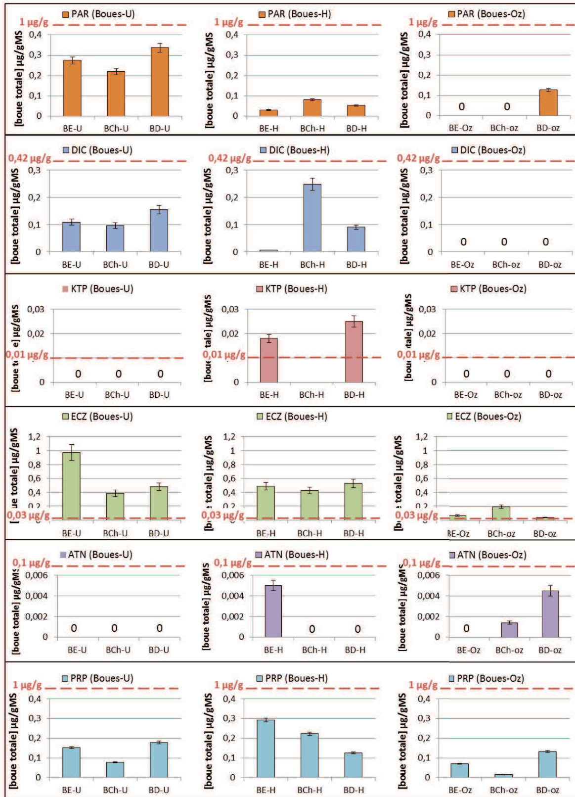
Figure 51 : Teneurs en médicaments dans les boues épaissies, chaulées et digérées et comparaison avec les concentrations de la littérature dans les boues secondaires (concentrations affichées par les traits rouges en pointillés) (suite)
