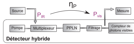
FIGURE 2.18 – Schéma de principe de la mesure du rendement global de conversion
