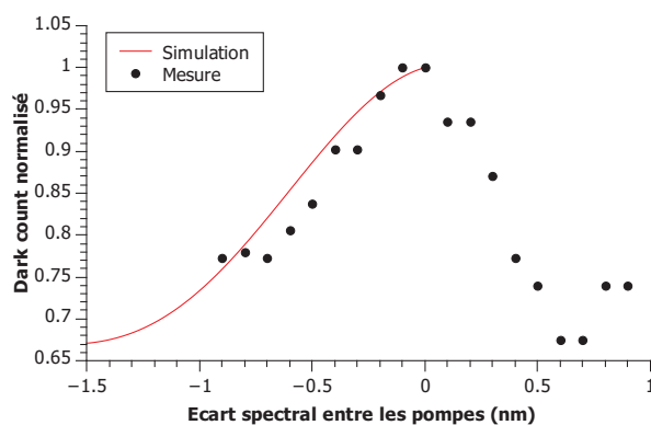
FIGURE 4.11 – Évolution du dark count optique en fonction de l'écart spectral entre les deux raies de pompe.
