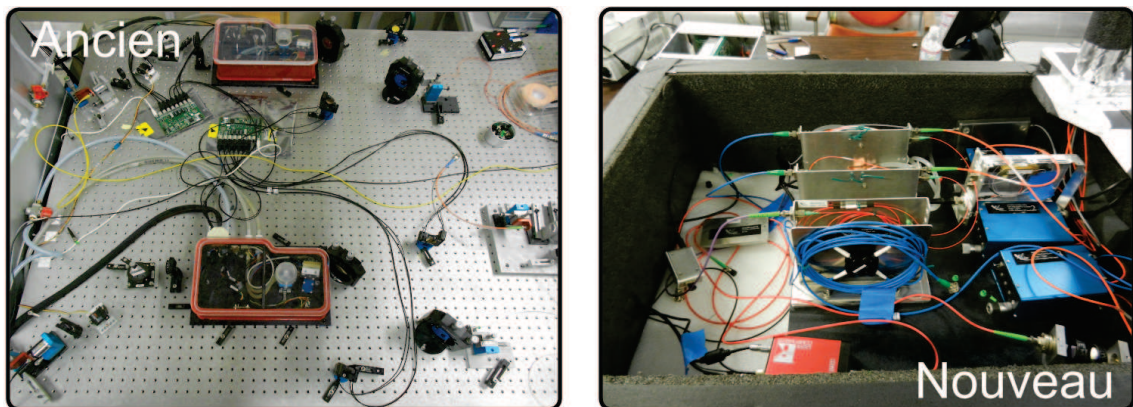
FIGURE 7.2 – Le nouveau banc ne nécessite aucun réglage sur marbre, il est beaucoup plus compact et simple d'utilisation
