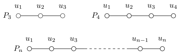
Figure 6: Les graphes P_3 , P_4 et P_n sont appelés chemins de longueur respective 3, 4 et n .
