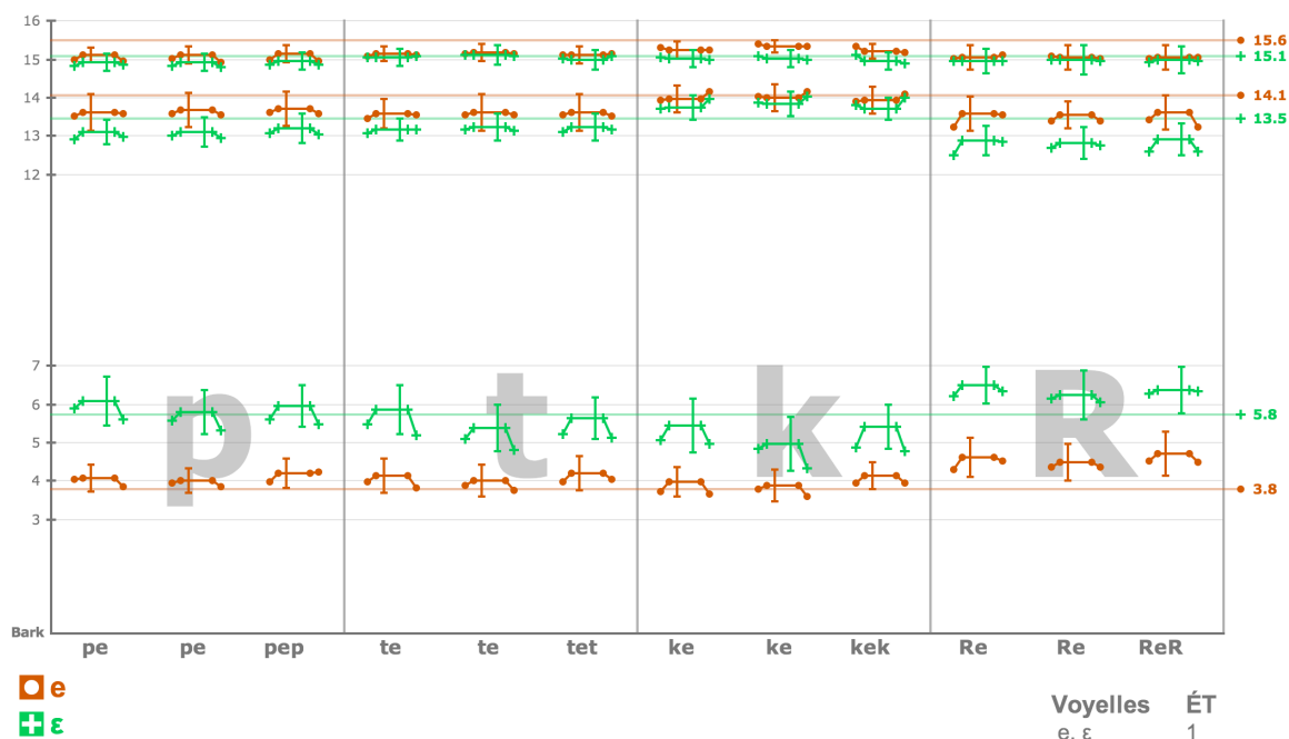
Figure 117 : Contraste acoustique entre les voyelles e/ε produites en contexte nul (traits horizontaux) et dans des logatomes CVCVCVC où C = [p, t, k, ʁ]. Valeurs de F1, F2 et F3 (en Bark) sont calculées à partir de 4 répétitions par 10 Françaises natives et relevées à un tiers, à la moitié et 2 tiers de la voyelle. L'écart type tracé est de 1
