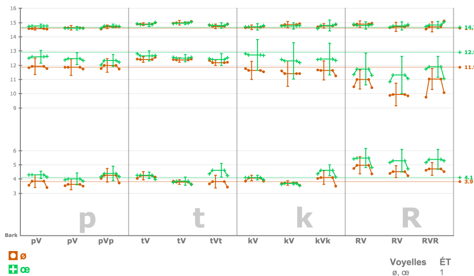
Figure 146 : Valeurs moyennes de F1, F2 et F3 (en Bark) de ø/œ produit par la locutrice T9 en contexte nul (traits horizontaux) et dans des logatomes CVCVCVC où C = [p, t, k, ʀ], calculées à partir de 10 répétitions. Valeurs relevées à un tiers, à la moitié et à deux tiers de la durée vocalique. L'écart type tracé est de 1. L'écart type tracé est de 1. Notons la différence de valeurs de F1 et/ou F2 en isolation et en syllabe finale tVt
