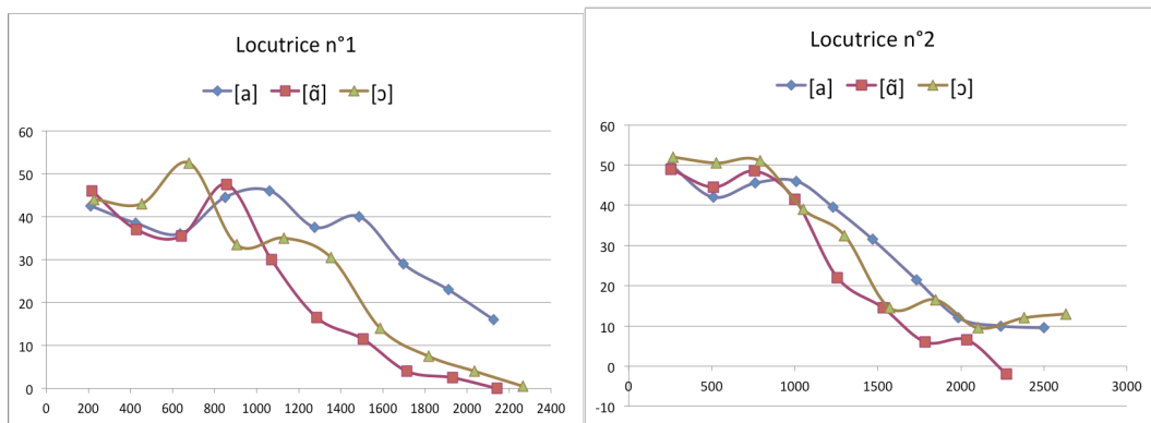
Figure 83: Valeurs en Hertz (abscisses) et en dB SPL (ordonnées) des 10 premiers harmoniques pour les voyelles [ɔ]-[ã]-[a] pour la locutrice n°1 (gauche) et la locutrice n°2 (droite). Moyenne de 2 exemplaires de la locutrice pour chaque voyelle.
