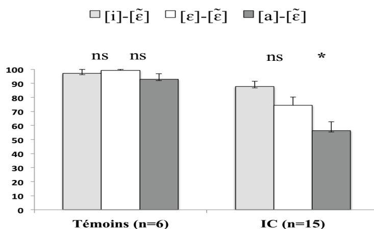
Figure 65: Détection de la voyelle [ê] parmi les voyelles [i], [ɛ] et [a]. Test PLSD de Fisher avec * si p < 0,05 .
