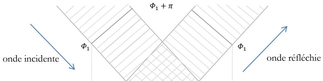
Figure 3.21 : Représentation géométrique de la réflexion (incidence oblique) d'une onde OAM sur une surface plane.
