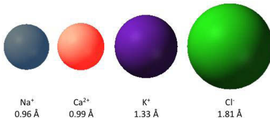
Figure 14 : Rayons ioniques 46
