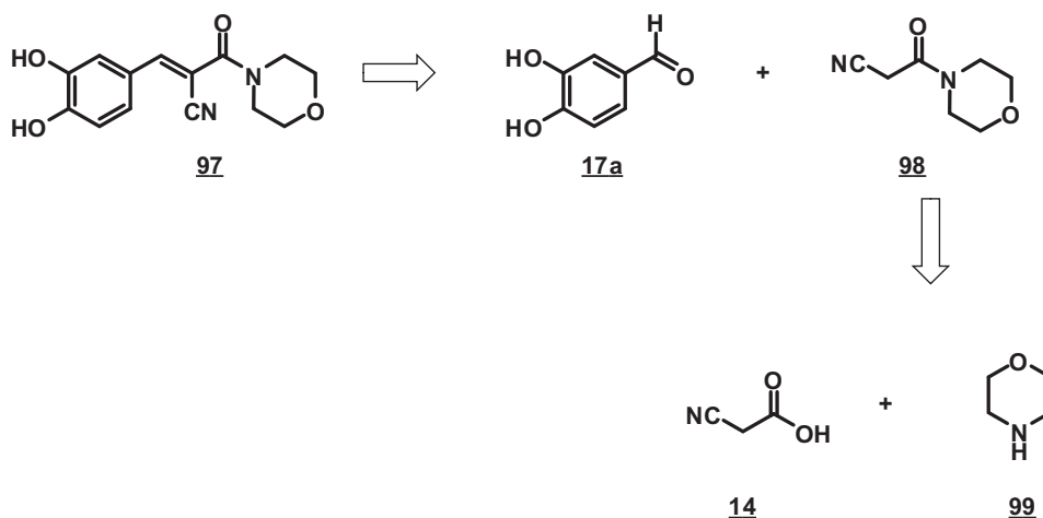
Schéma 34 : Rétrosynthèse de l'amide 96
