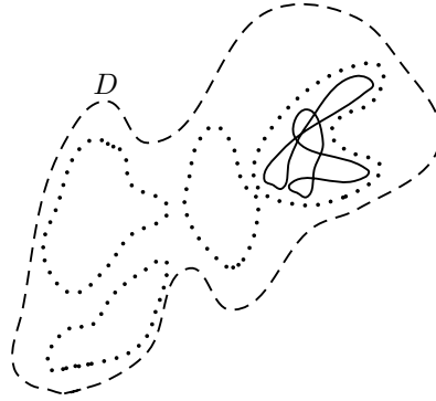
Fig. 1.1. : Représentation de quatre boucles CLE_\kappa en pointillés et des boucles browniennes en traits pleins à l'intérieur d'une d'elles.
