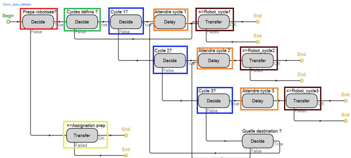
Figure 8.24 : Vue du processus « Choix_mode_prepa »
