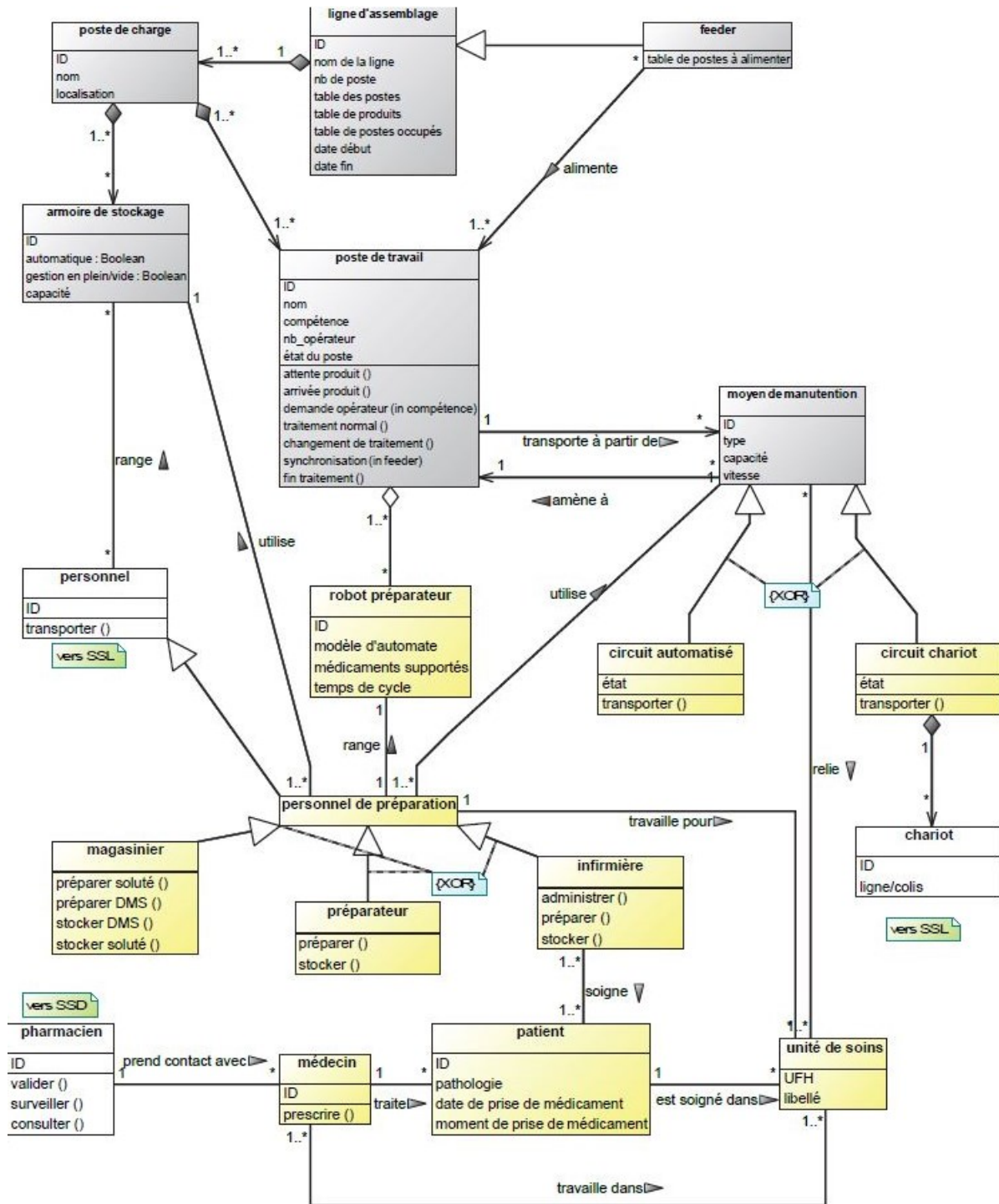
Figure 6.32 : Sous-système Physique conçu par [HUET 11]
