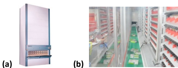
Image 1.1 : (a) Stockeur rotatif vertical (b) stockeur avec tapis
