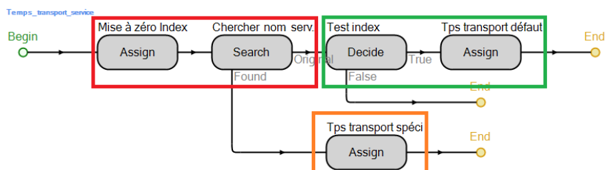
Figure 8.39 : Vue du processus recherchant le temps de transport des demandes
