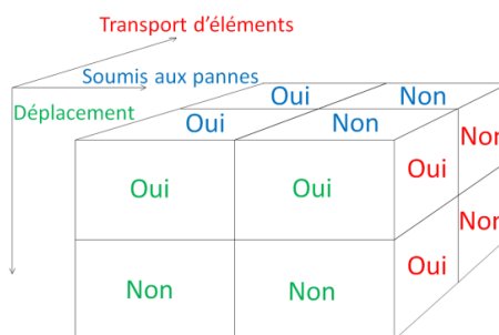
Figure 7.28 : Matrice cubique de sélection du type d'acteur sous SIMIO
