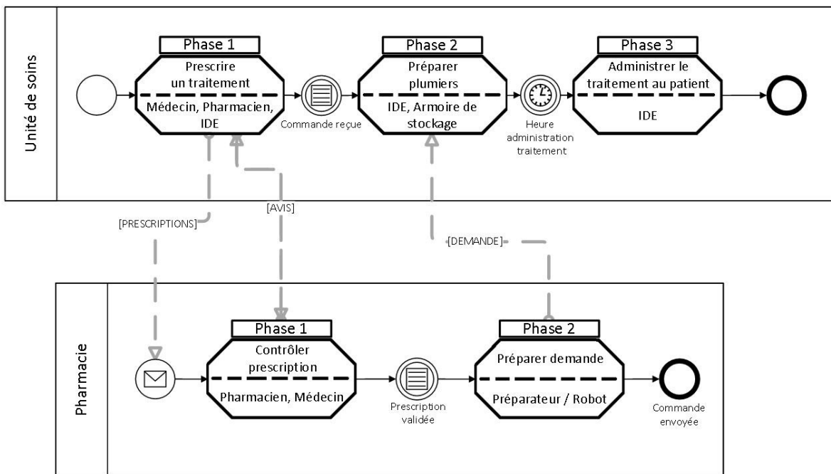
Figure 6.28 : Exemple d'application du formalisme macroscopique
