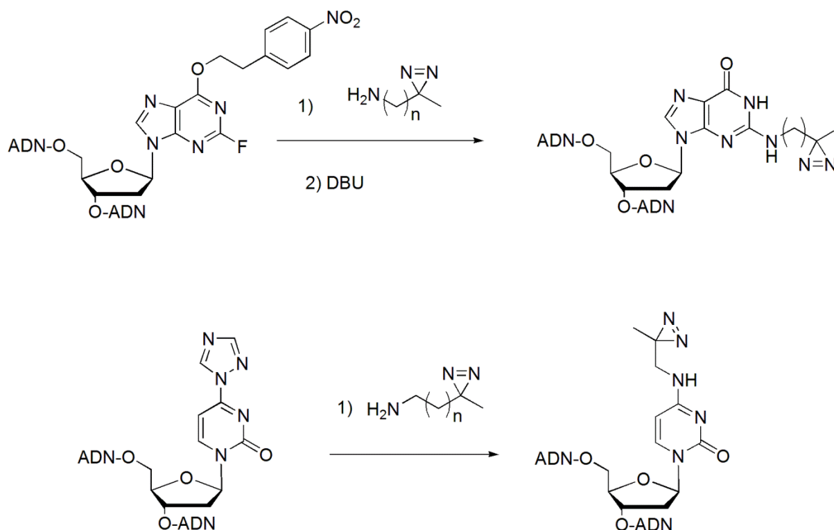
Figure 106. Fonctionnalisation post-synthétique de la 2-Fluoro-2'-désoxyinosine et de l'O 6 -triazolyl-2'-désoxyuridine par des diazirines aliphatiques.
