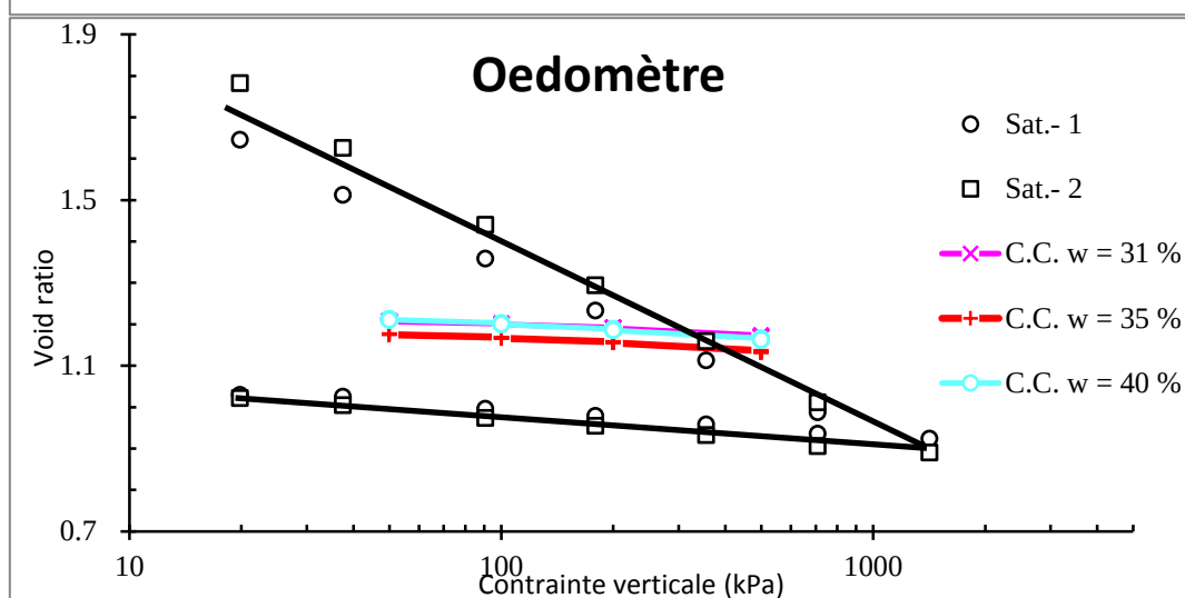
Figure II - 116 : Indice des vides en fonction de la contrainte verticale
