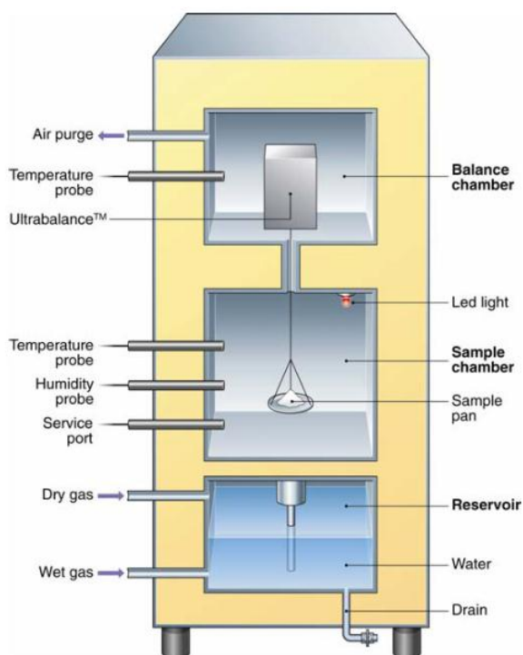
Figure III - 24 : Schéma et photo de l'appareil DVS Intrinsic (DVS Intrinsic Brochure)
