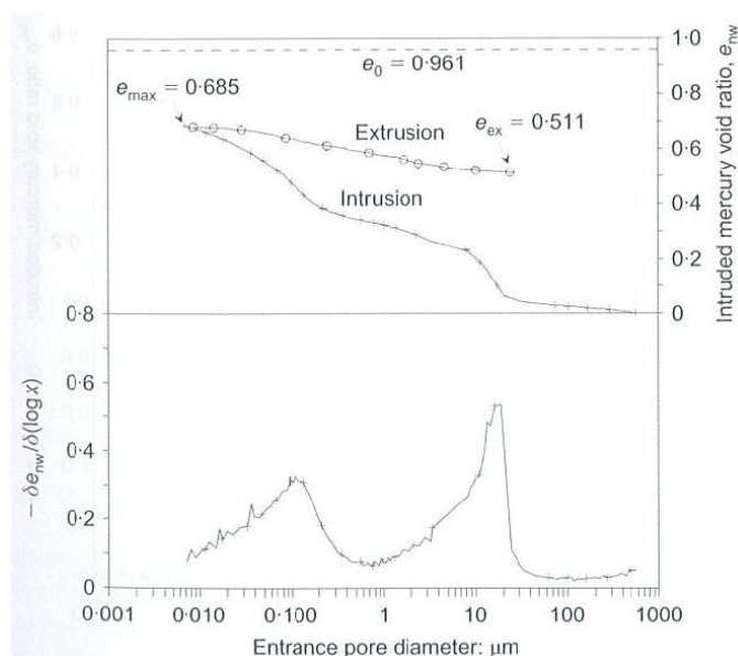
Figure II - 48 : Distribution des tailles des pores pour l'argile Londres (après MONROY et al., 2010)
