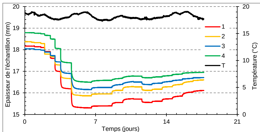
Figure I - 15 : Evolution de l'épaisseur pour les échantillons compactés à l'optimum (sous une succession de charge de 1-2-5-10-20-40-80-40-20-10-5-2-1 kg)
