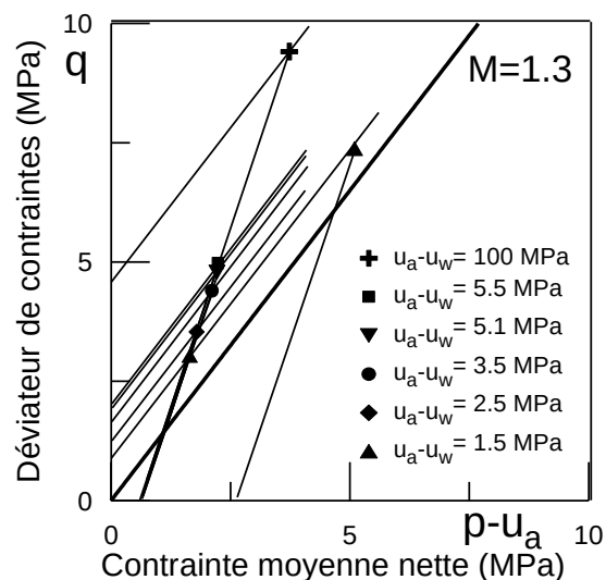
Figure IV - 20 : Lignes d'état critique du limon de Jossigny à fortes contraintes et moyennes à fortes succions (FLEUREAU et al., 1998)
