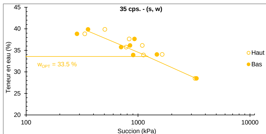
Figure II - 79 : Succions mesurées par papier filtre (s - w) pour les échantillons compactés avec l'énergie de 35 coups/couche
