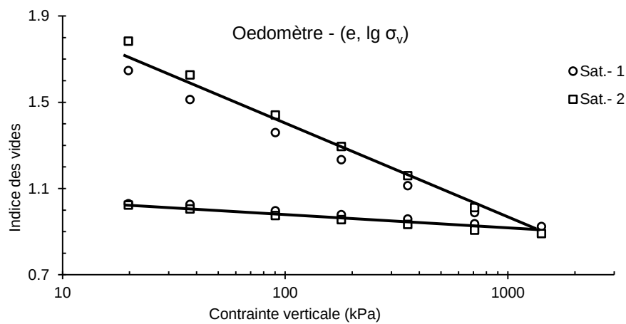
Figure I - 14 : Variation de l'indice des vides en fonction de la contrainte verticale en coordonnées semi-logarithmiques
