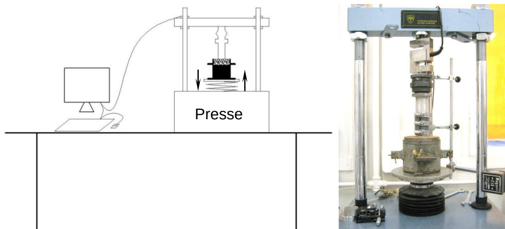
Figure II - 53 : Le dispositif expérimental de 2012 pour tester l'orniérage
