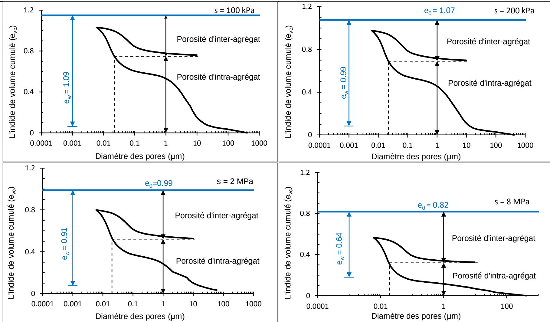
Figure II - 123 : Courbes de porosimétrie en indice de volume cumulé pour les échantillons compactés avec succion contrôlées (100 kPa, 200 kPa, 2 MPa, 8 MPa)
