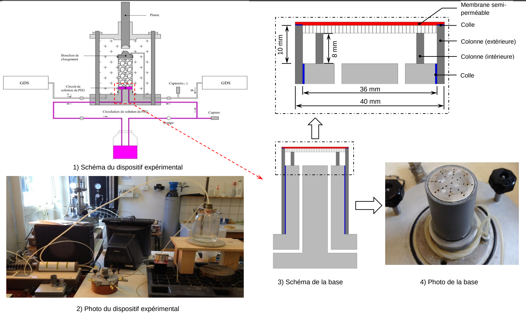
Figure IV - 41 : Montage de l'essai triaxial avec la technique osmotique
