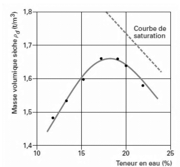
Figure II - 8 : Courbe PROCTOR du Limon de Jossigny (DELAGE et CUI, 2000)
