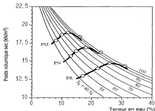
Figure II - 7 : Courbe PROCTOR d'une argile avec différentes énergies de compactage (d'après SERRATRICE, 1995)
