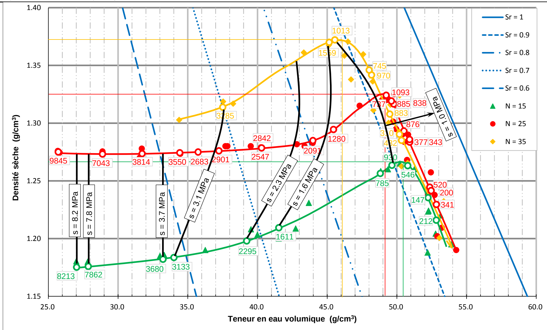
Figure II - 86 : Courbe d'iso-succion du sol compacté ( \theta , \rho_d )
