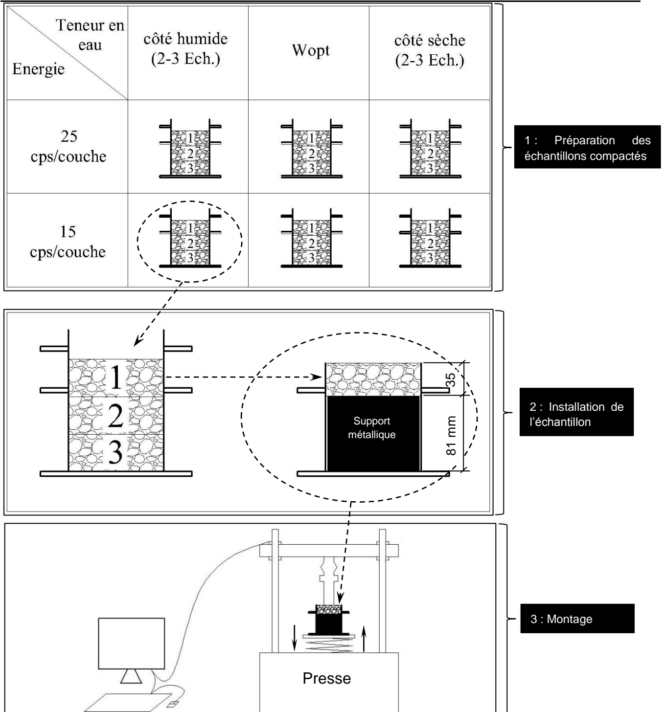
Figure II - 54 : Schéma de la procédure expérimentale pour le test d'orniérage en utilisant le dispositif de 2012
