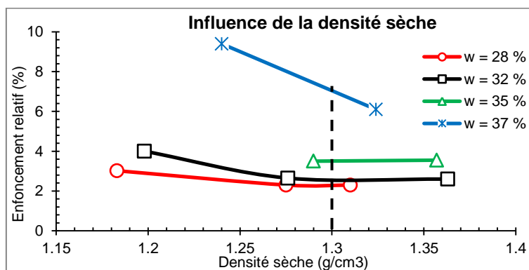
Figure II - 111 : Influence de la densité sèche sur l'enfoncement relatif (≈ 30000 cycles)
