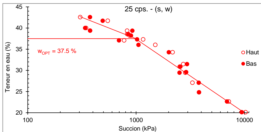
Figure II - 78 : Succions mesurées par papier filtre (s - w) pour les échantillons compactés avec l'énergie de 25 coups/couche (côté sec + côté humide)
