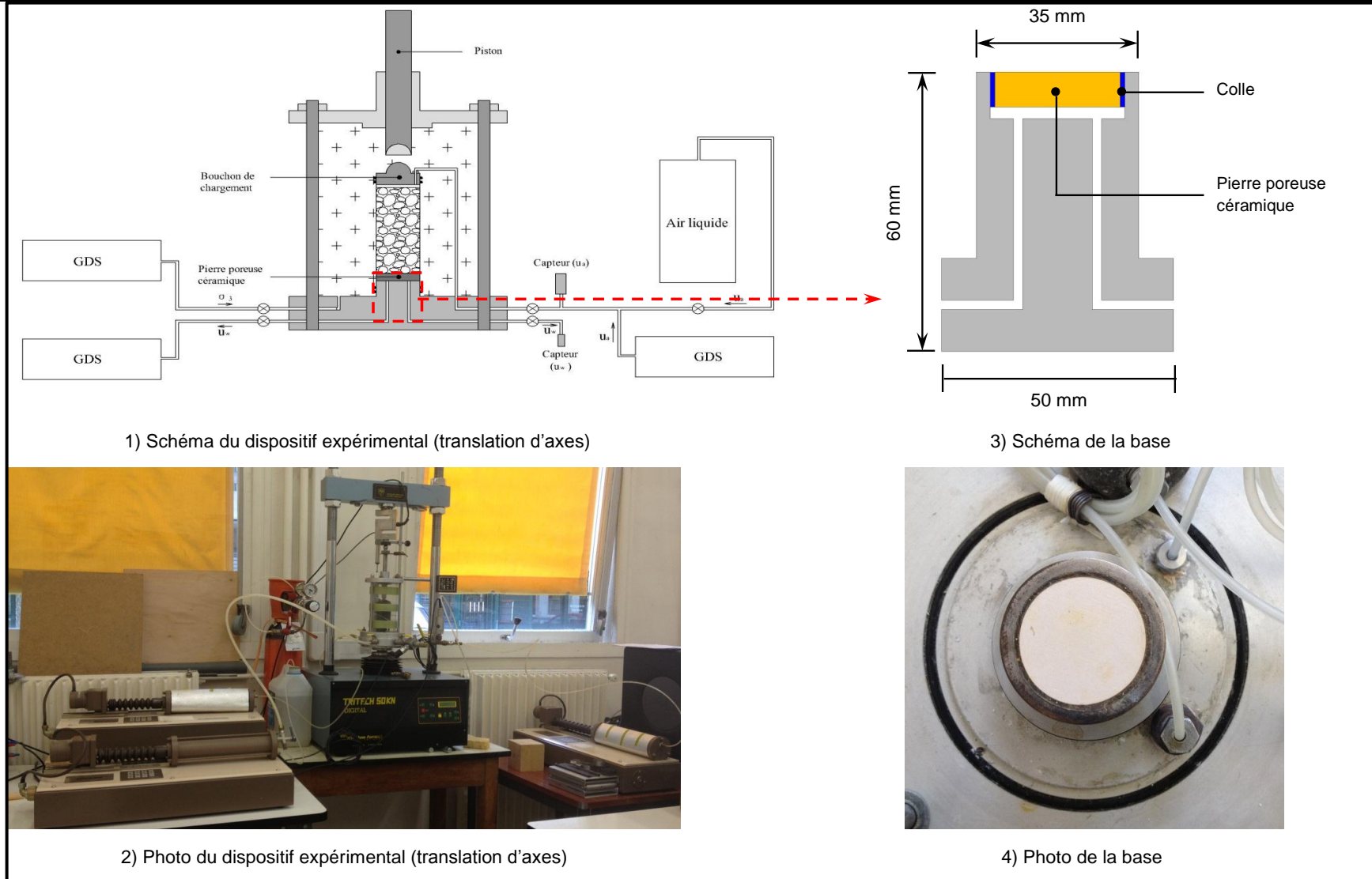
Figure IV - 28 : Montages construits pour l'essai triaxial avec la technique de translation d'axe
