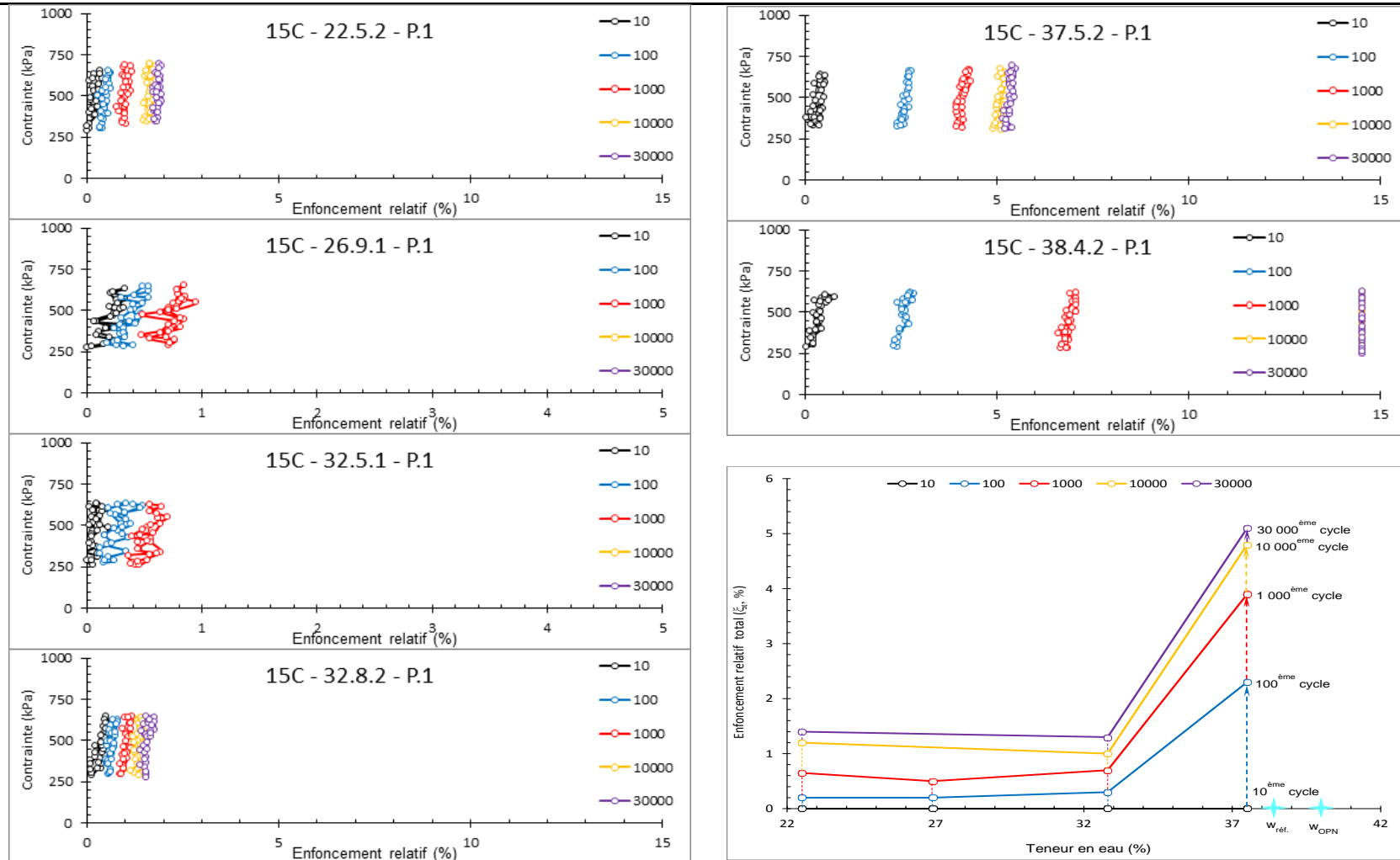
a) Contrainte en fonction de l'enfoncement relatif
