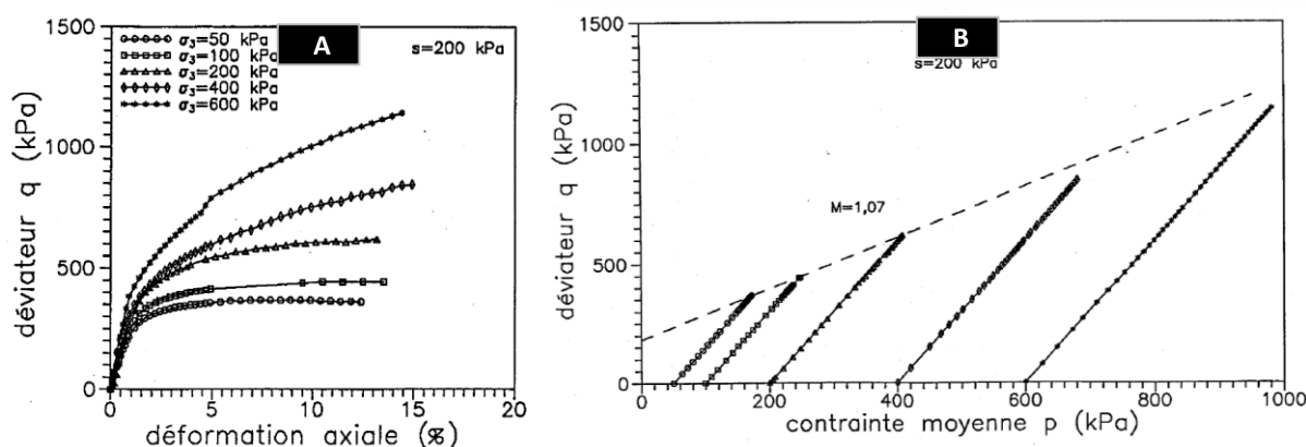
Figure IV - 16 : Cisaillement à \sigma_3 = 50 kPa et surface de chargement (d'après CUI, 1993)
