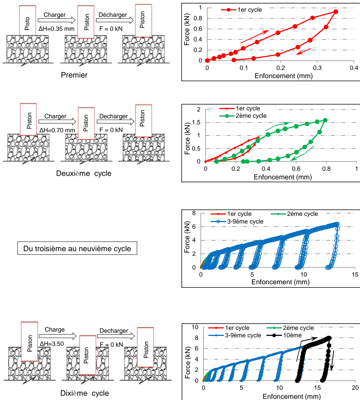
Figure II - 56 : Schéma du deuxième type de chargement pour le test d'orniérage en utilisant le dispositif de 2012
