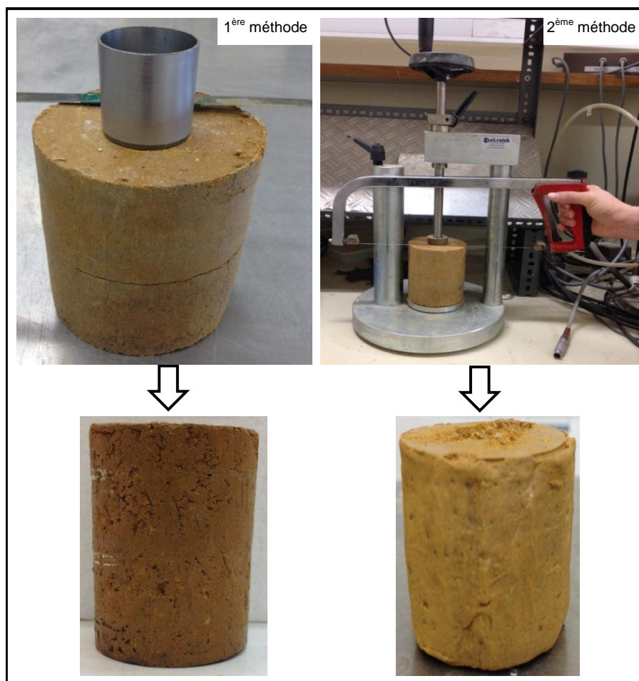
Figure I - 25 : Deux méthodes de la fabrication des éprouvettes pour les essais traxiaux compactés (1 ère : par une carottier ; 2 ème : par une machine et une lame de fer)
