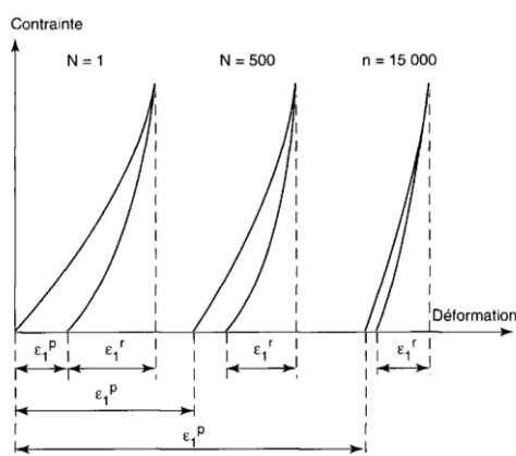
Figure II - 29 : Evolution des cycles contraintes/déformations au cours des chargements (d'après PAUTE et al., 1994)
