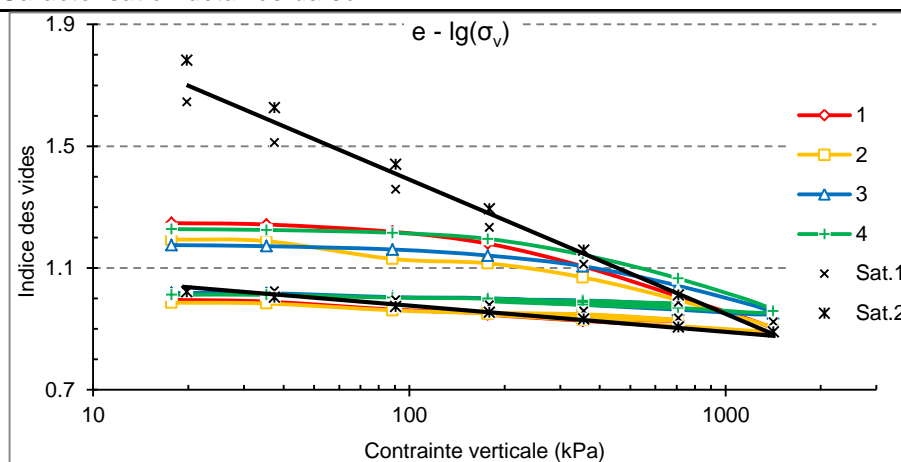
Figure I - 16 : Indice des vides en fonction de la contrainte verticale pour les échantillons saturés et compactés à l'optimum
