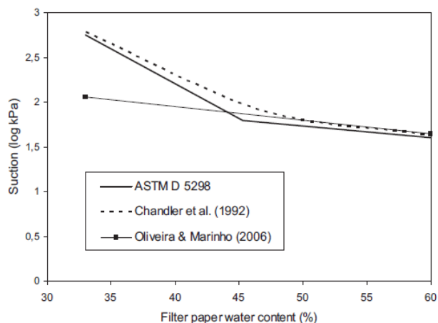
Figure II - 14 : Un résumé sur les courbes d'étalonnage du papier filtre Wateman No. 42 réalisé par différents auteurs et la comparaison (d'après BICALHO et al. ; 2007)
