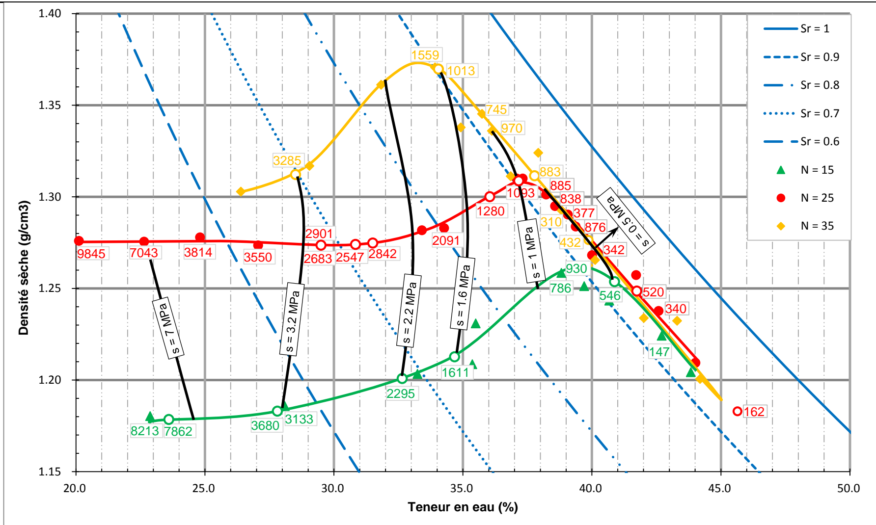
Figure II - 85 : Courbe d'iso-succion du sol compacté ( w , \rho_d )
