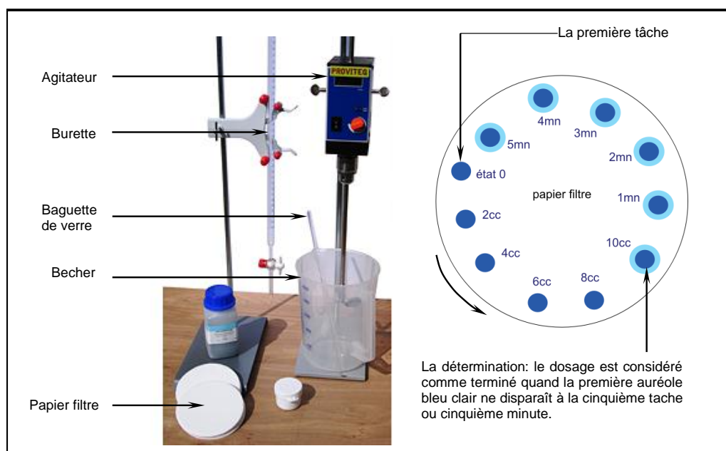
Figure I - 4 : L'appareillage et le test à la tache de l'essai au bleu de méthylène (source internet)
