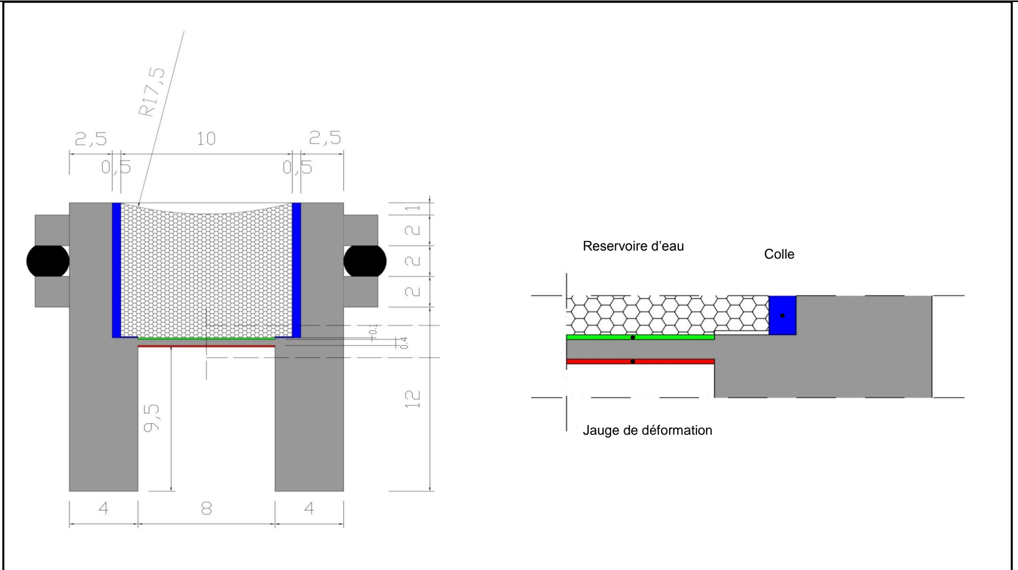
Figure A.I - 6 : Schéma du tensiomètre haute capacité à l'ECP
