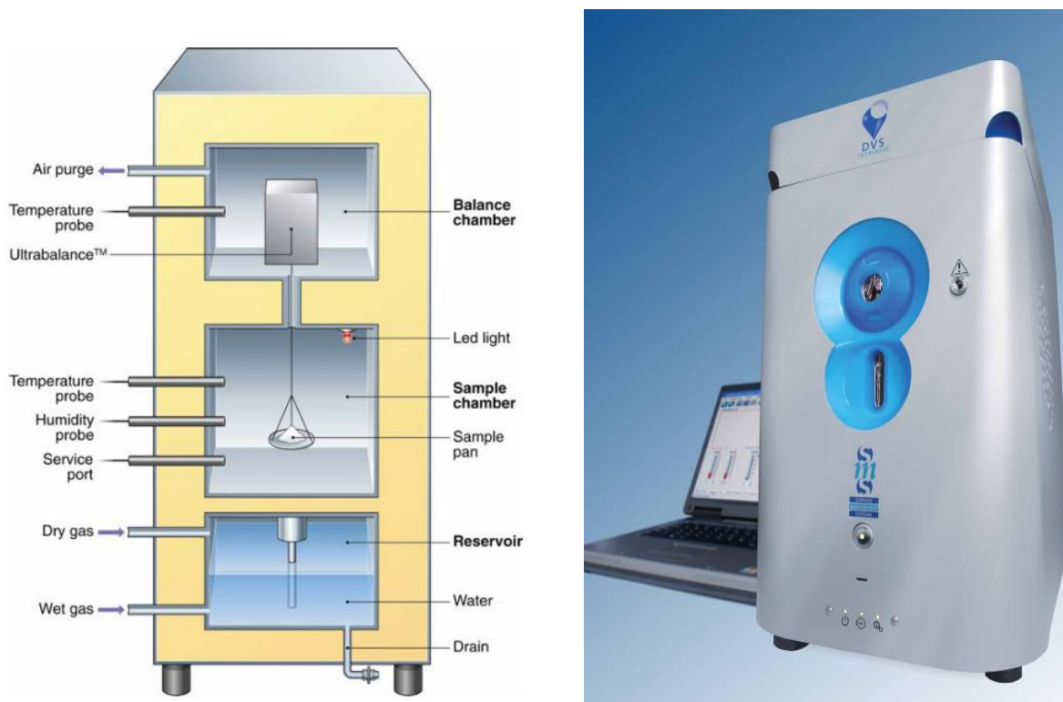
Figure III - 24 : Schéma et photo de l'appareil DVS Intrinsic (DVS Intrinsic Brochure)
