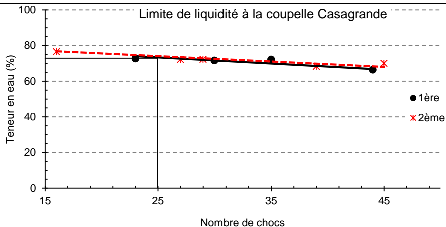
Figure I - 2 : Détermination de la limite de liquidité à la coupelle de Casagrande
