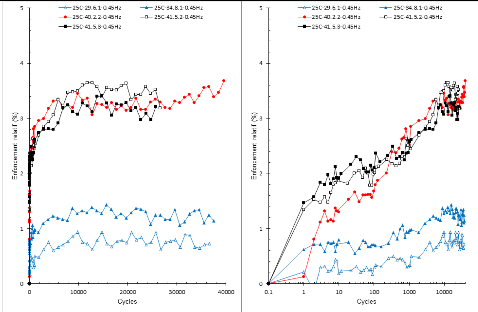
Figure II - 105 : Résultats d'enfoncement relatif en fonction du nombre de cycles du programme 2, 25 cps.
