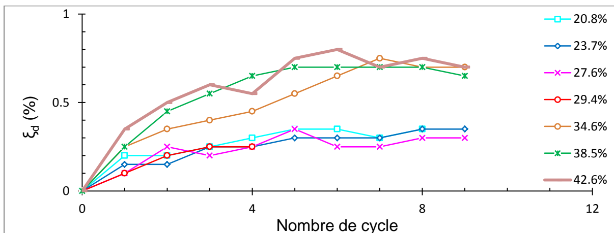
Figure II - 93 : Enfoncement relatif différé (ξ d ) en fonction du nombre de cycles (25 cps.)
