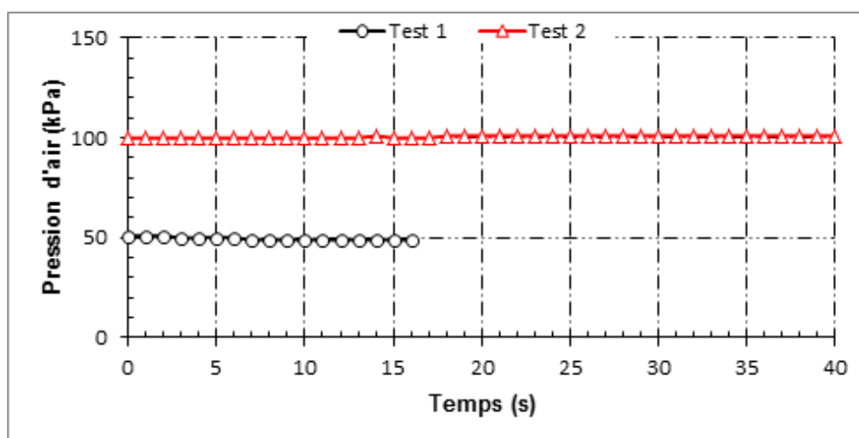
Figure II - 71 : Le test d'étanchéité du montage pour la mesure de perméabilité à l'air
