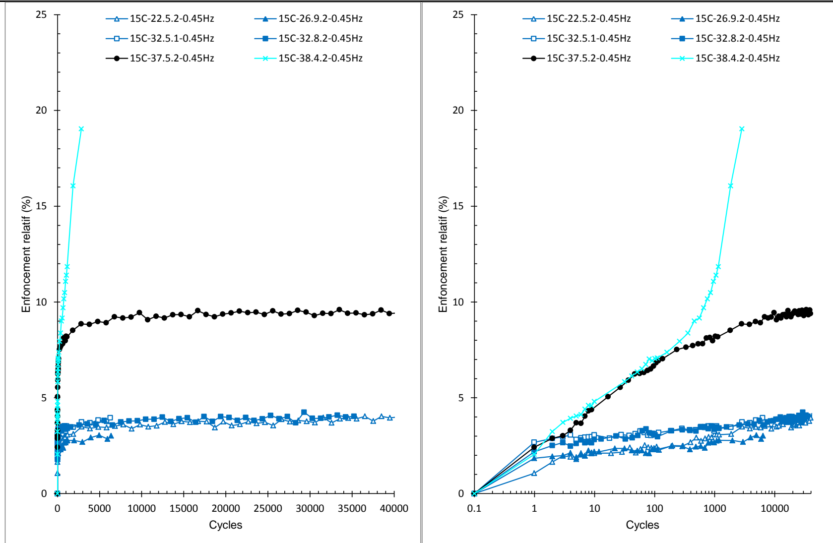
Figure II - 98 : Résultats d'enfoncement relatif en fonction du nombre de cycles du programme 1, 15 cps.
