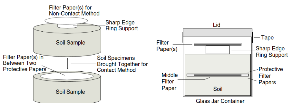
Figure II - 12 : La mesure de succion pour les sols compactés (d'après BULUT, 2001)
