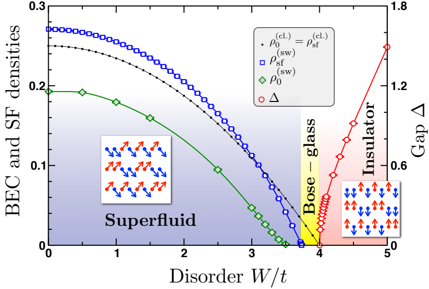
Figure 4: Evolution des extrapolations à la limite thermodynamique de la densité superfluide \rho_{\text{sf}} , la densité du condensat de Bose-Einstein \rho_0 et le gap dans le spectre des excitations \Delta avec la force du désordre W/t . Les densités classiques ( \bullet ) sont égales et s'annulent au bord de la bande W = 4t . Les quantités corrigées par les ondes de spin \rho_{\text{sf}}^{(\text{sw})} ( \square ) et \rho_0^{(\text{sw})} ( \diamond ) s'annulent à des points différents W_0 < W_{\text{sf}} < 4t , laissant place à une phase gapless verre de Bose (BG) sur une fenêtre finie du désordre, avant l'apparition de l'isolant gappé pour W > 4t . Les vignettes montrent les phases superfluide et isolantes dans la représentation des pseudo-spins. Les moyennes sur le désordre ont été faites sur plusieurs centaines d'échantillons désordonnés. La ligne verte est un guide visuel.
