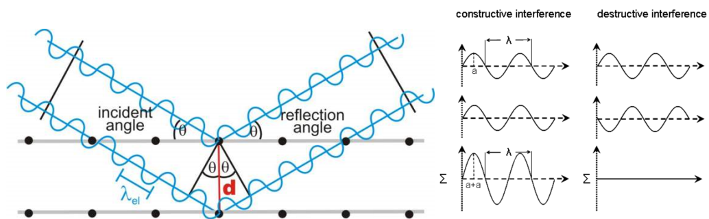
Figure 3-1 A gauche : schéma illustrant la loi de Bragg (les points noirs représentent les atomes des plans). A droite : illustration du phénomène d'interférence constructive et destructive.
