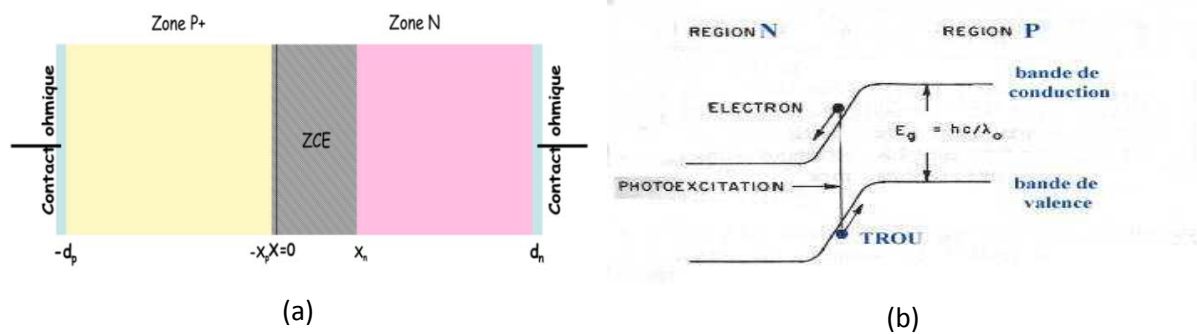
Fig.3.6. Structure (a) et diagramme de bande (b) d'une cellule photovoltaïque.
