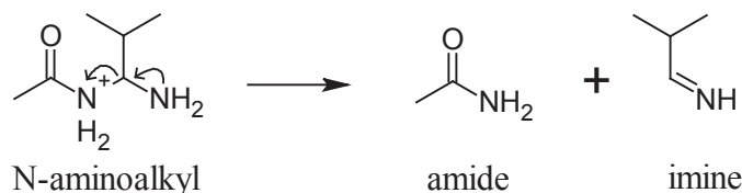
Schéma 31 : Décomposition du motif gem-diaminoalkyl en milieu acide
