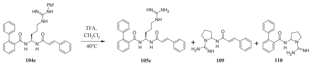
Schéma 30 : Sous-produits issus de la déprotection de l'arginine en milieu acide
