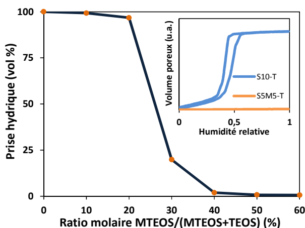
Figure II.18. Prise en eau à RH = 100% de films mésoporeux calcinés à 450°C en fonction du ratio molaire MTEOS/TEOS. En insert, les isothermes d'adsorption et désorption d'eau obtenues par éllipsométrie porosimétrie environnementale pour un film de SiO 2 pure (100 mol% TEOS, S10-T) et un film hybride méthylé de SiO 2 (50 mol% MTEOS/50 mol% TEOS, S5M5-T) calcinés à 450°C, 10 min.
