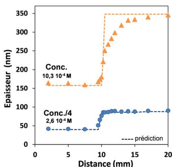
Figure I.14. Épaisseur des films mésoporeux d'oxyde de titane (points expérimentaux et droites théoriques) en fonction de la concentration en précurseur non volatil des solutions. Les points sont obtenus à 60°C avec un profil de vitesse composé de deux paliers à vitesse constante de 1 mm.s -1 et 6 mm.s -1 .
