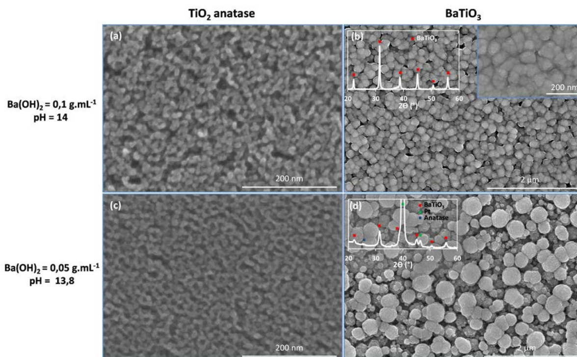
Figure IV.16. Clichés de FEG-SEM d'un film T^M sur alumine avant (a, c) et après (b, d) traitement hydrothermal dans des solutions de Ba(OH)_2 à 0,1 \text{ g.mL}^{-1} et 0,05 \text{ g.mL}^{-1} avec en insert les diffractogrammes des rayons X des films correspondants.
