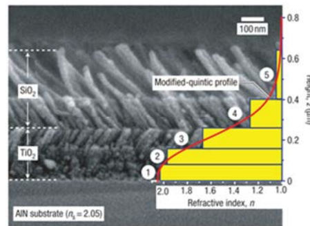
Figure II.4. Cliché SEM-FEG en coupe d'un film à gradient d'indice de réfraction obtenu par GLancing Angle Deposition (GLAD) et composé d'un empilement de 5 couches à base de TiO 2 et SiO 2 . 44
