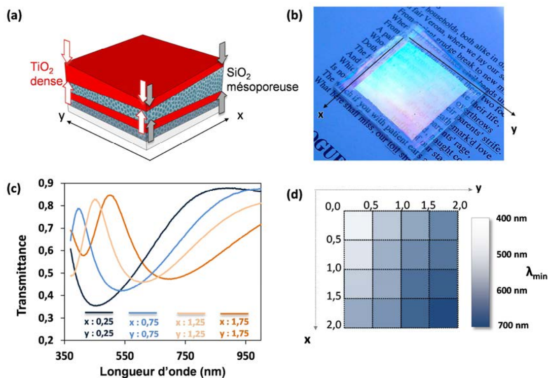
Figure I.17. (a) Illustration de l'empilement réfléchissant composé de couches de TiO 2 dense et SiO 2 mésoporeuse ayant un gradient bidirectionnel. (b) Photo de l'empilement multicouche déposé sur verre. (c) Spectres UV-visible en transmission à incidence normale du système multicouche pour différentes coordonnées dans le plan x-y. (coordonnée en centimètre). (d) Evolution de la longueur d'onde minimale de transmission en fonction des coordonnées x-y.
