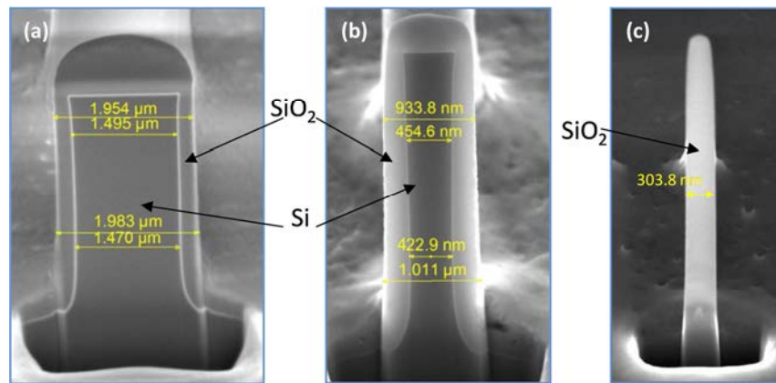
Figure IV.14. Clichés de MEB en coupe des nanofils de silicium de (a) 1,7 \mu\text{m} , (b) 700 nm et (c) 250 nm de diamètre usinés par sonde ionique focalisée après dépôt de la couche mésoporeuse de silice, imprégnation par l'agent vitrifiant, traitement thermique et lavage dans l'acide nitrique concentré.
