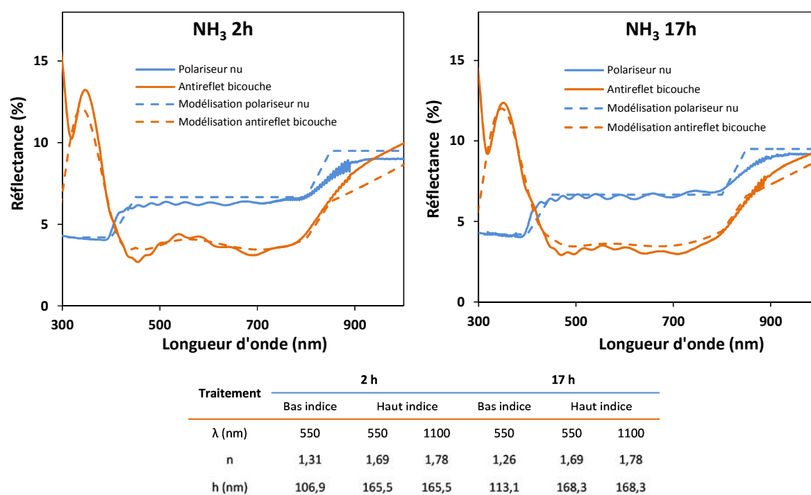
Figure II.38. Courbes de réflectance à incidence normale des polariseurs avec l'empilement antiréfléctif bicouche déposé sur une face du polariseur pour des temps de traitement en vapeur d'ammoniaque de 2 h et 17 h. Tableau des valeurs d'indices de réfraction et d'épaisseur des couches bas et haut indices utilisées pour les modélisations.
