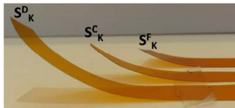
Figure IV.6. Photographie illustrant les différents rayons de courbures des films S_K^D , S_K^C et S_K^F à RH = 50%.
