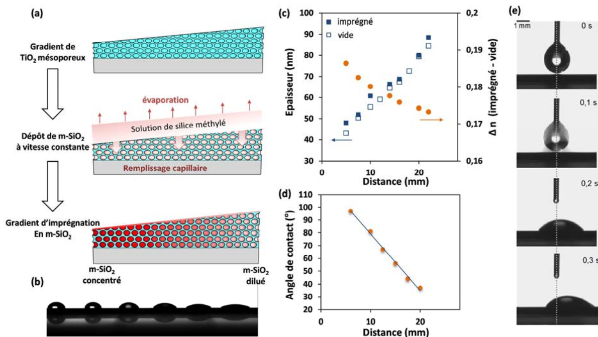
Figure I.18. (a) Schéma de la préparation de la surface à gradient de mouillabilité. (b) Photo des gouttes d'eau déposées à différentes distances. (c) Courbe de l'épaisseur de la couche mésoporeuse de \text{TiO}_2 avant et après imprégnation en fonction de la distance et courbe représentant la différence d'indice de réfraction entre la couche imprégnée et la couche mésoporeuse vide en fonction de la distance. (d) Valeurs des angles de contact en fonction du gradient de mouillabilité. (e) Séquence photographique montrant le mouvement d'une goutte sur une surface à gradient de mouillabilité.
