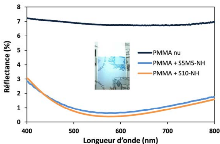
Figure II.35. Spectres de réflectance dans le visible à incidence normale pour les films S5M5-NH et S10-NH déposés sur les deux faces du substrat de PMMA. En insert, une photographie de l'antiréflex S5M5-NH.
