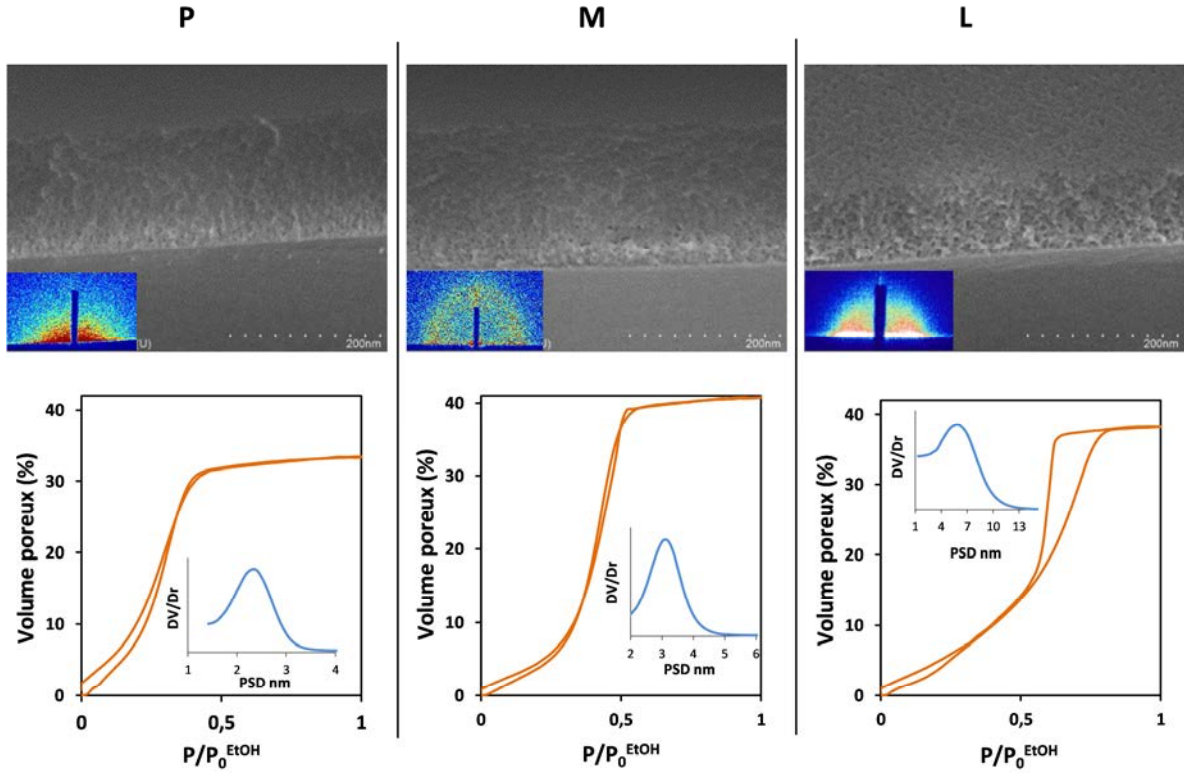
Figure III.2. Images SEM-FEG en coupe, clichés de GI-SAXS et isothermes correspondants d'adsorption et désorption d'éthanol obtenus par EEP (en insert les distributions de taille de pore) des films P, M et L.
