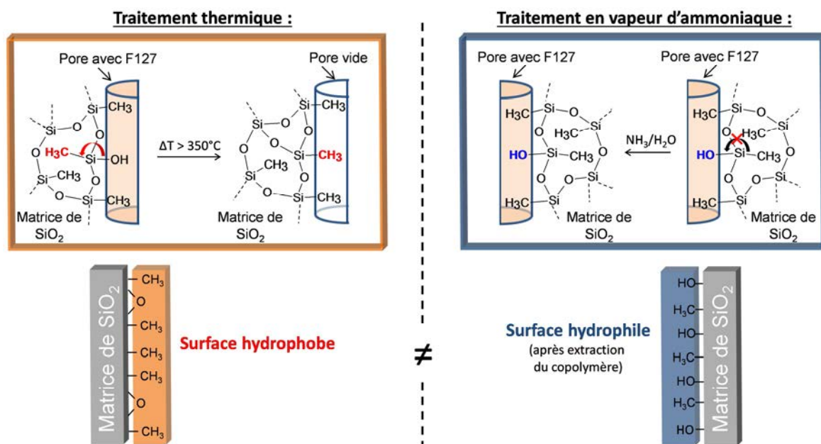
Figure II.26. Schéma illustrant le changement de conformation du motif \text{Me-Si}(\text{O})_3^- à l'interface du réseau inorganique et d'un pore générant la propriété hydrophobe de S5M5-T et partiellement hydrophobe de S5M5-N.
