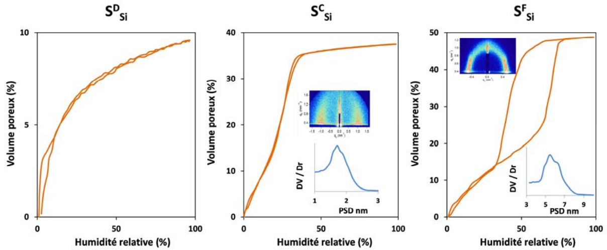
Figure IV.3. Isothermes d'adsorption et désorption d'eau obtenus par EEP (en insert les distributions de taille de pore) des films S^D_{Si} , S^C_{Si} et S^F_{Si} et les clichés de diffusion obtenus en GISAXS correspondants.
