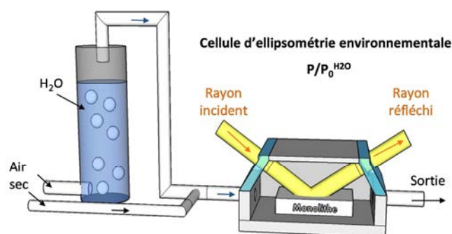
Figure III.15. Illustration du montage d'ellipsométrie environnementale.
