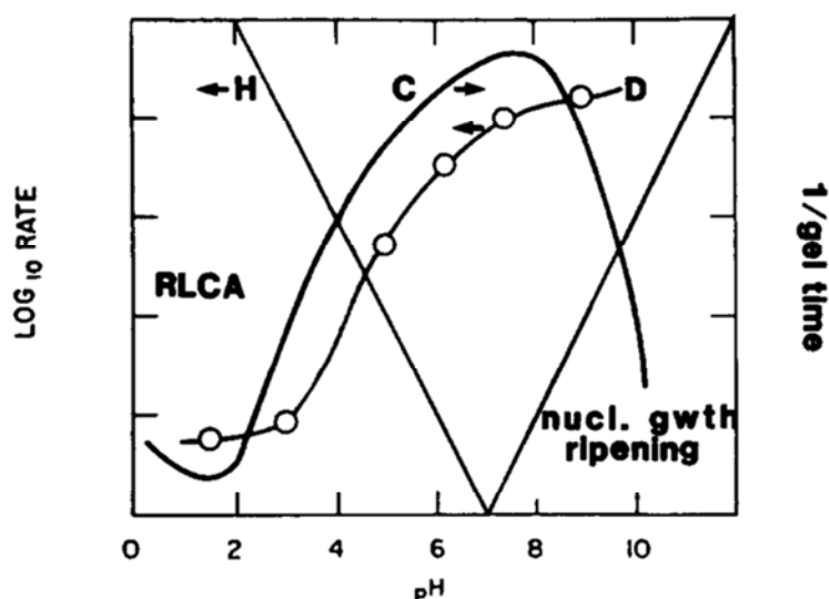
Figure 1.2. Cinétiques d'hydrolyse (H), condensation (C) et dissolution (D) d'un système à base de TEOS, pour un taux d'hydrolyse fixé arbitrairement, en fonction du pH. 1
