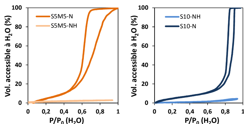
Figure II.34. Isothermes d'adsorption et désorption d'eau des films S5M5-N, S5M5-NH, S10-N et S10-NH obtenus par EEP.
