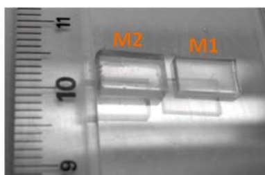
Figure III.14. Monolithes de xérogel de silice fonctionnalisée par des groupes amines transparents d'une épaisseur de 1 mm et 2 mm.
