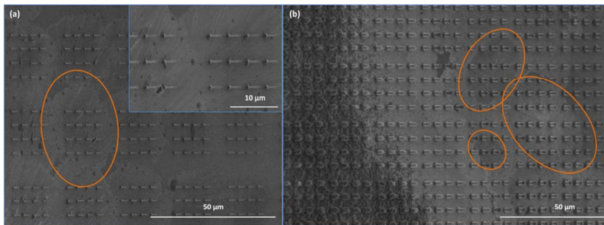
Figure IV.12. Clichés de MEB des nanofils de silicium de (a) 350 nm et (b) 1,7 µm de diamètre après dépôt de la couche mésoporeuse de silice, imprégnation par l'agent vitrifiant, traitement thermique et lavage dans l'acide nitrique concentré.
