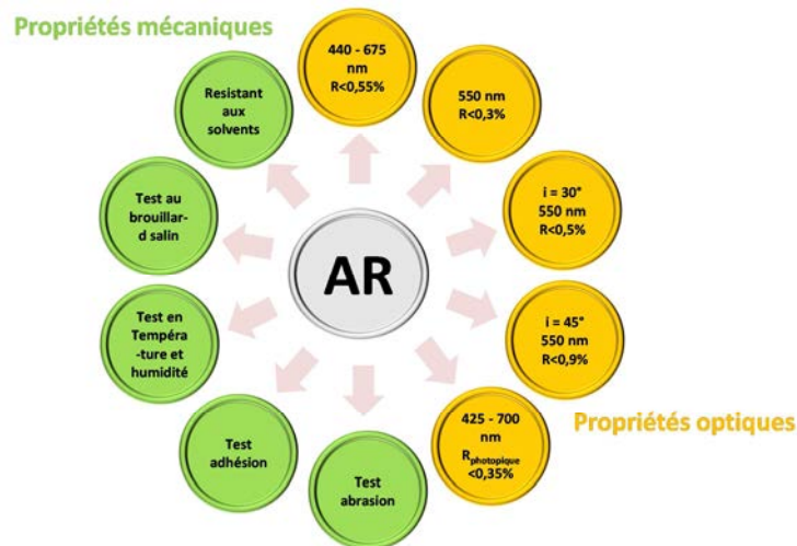
Figure II.15. Schéma reprenant les principaux tests mécaniques et propriétés optiques à valider pour qualifier l'antireflet.
