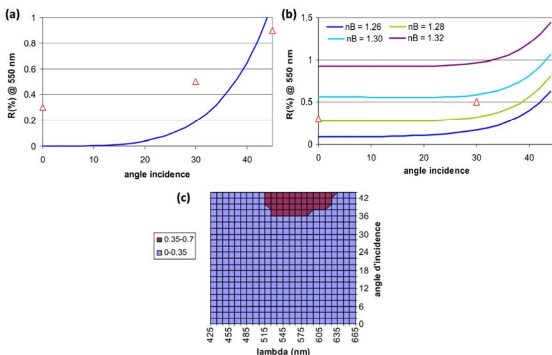
Figure II.17. (a) Valeurs de réflectance simulées à différents angles d'incidence sur substrat de TAC ( n_{\text{substrat}} = 1,52 ) à \lambda = 550 nm pour un antireflet interférentiel monocouche ( n = 1,23 ). (b) Valeurs de réflectance simulées à différents angles d'incidence sur substrat de TAC ( n_{\text{substrat}} = 1,52 ) à \lambda = 550 nm pour des antireflets bicouches composés de n_{\text{haut indice}} = 1,65 et différents bas indices ( n_{\text{B}} ), les épaisseurs de couches n'ont pas été optimisées. Les triangles rouges représentent les limites imposées par le CdC. (c) Diagramme des valeurs de réflectance phototype pour un antireflet bicouche composé de n_{\text{haut indice}} = 1,65 et n_{\text{bas indice}} = 1,28 .
