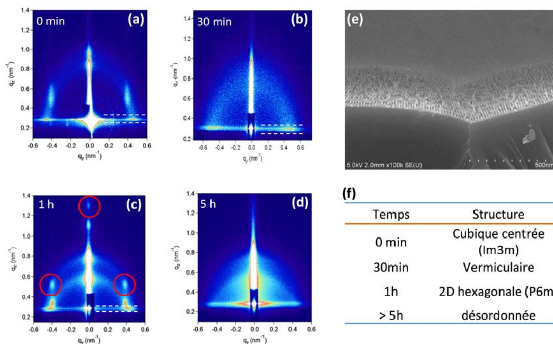
Figure II.28. (a-d) Clichés de diffraction GI-SAXS des films S10-N pour différents temps de TVA avec (f) les mésostructures correspondantes. Les cercles rouges correspondent aux signaux fantômes causés par les ondes évanescentes. 116 (e) Image de SEM-FEG d'un S10-N traité pendant 1 h présentant une structure 2D hexagonale.
