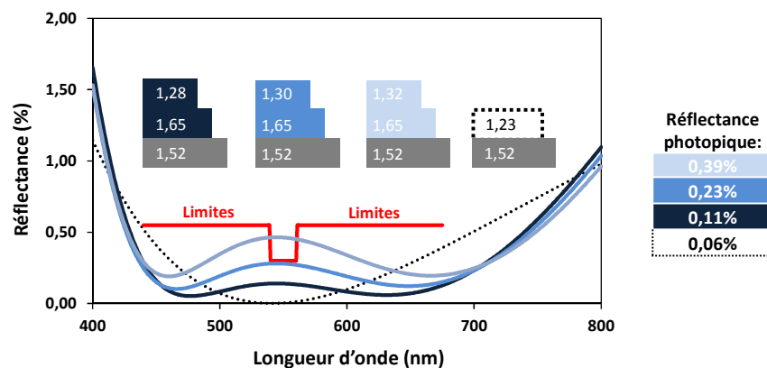
Figure II.16. Valeurs de réflectance simulées sur substrat de TAC ( n_{\text{substrat}} = 1,52 ) pour trois empilements interférentiels avec des épaisseurs h de (0,5\lambda)/n_{\text{haut}} indice pour les couches haut indice et (0,25\lambda)/n_{\text{bas}} indice pour les couches bas indice et un antireflet interférentiel monocouche. Avec \lambda = 550 nm. Le tracé rouge représente les limites de réflectance imposées par le cahier des charges.
