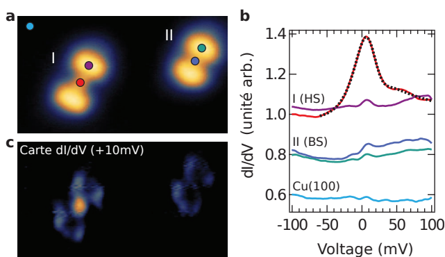
Figure X. – Spectroscopie sur des molécules de Fe-phen. a , Topographie montrant deux différentes conformations de Fe-phen sur Cu(100). b , Spectres dI/dV mesurés au centre et sur les lobes des molécules présentées en a . c , Carte dI/dV qui montre que la résonance est spatialement localisée au niveau de l'ion de fer de la molécules dans la conformation I. Les images ont une taille de 6.7 nm × 2.7 nm.
