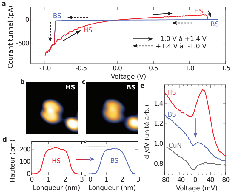
Figure XIII. – Commutation de l'état de spin et l'état de conduction d'un molécule de Fe-phen sur une surface de CuN/Cu(100). a , Courbe I(V) mesurée sur une molécule unique. La courbe montre deux états de conduction avec une hystérèse. Topography de la molécule sondée lorsqu'elle est dans l'état de b , haute conduction et c , basse conduction. Les topographies suggèrent que la molécule est dans b , l'état haut spin et c , l'état bas spin, respectivement. d , Profils de hauteur de la molécule représentée dans les topographies b et c . e , Spectres dI/dV de la molécule lorsqu'elle est dans l'état de haute et basse conduction. Toutes ces données permettent d'attribuer l'état de haute conduction (basse conduction) à l'état haut spin (bas spin). Les images ont une taille de 3.7 nm \times 3.7 nm.
