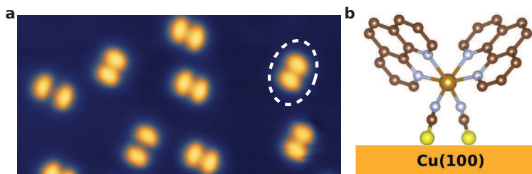
Figure VII. – Molécules de Fe-phen sur une surface de Cu(100). a , Topographie d’une sous monocouche de Fe-phen sur Cu(100) obtenue à 4 K. L’image a une taille de 17 nm × 8.5 nm. b , Schéma de la géométrie d’adsorption de la molécule de Fe-phen sur Cu(100).
