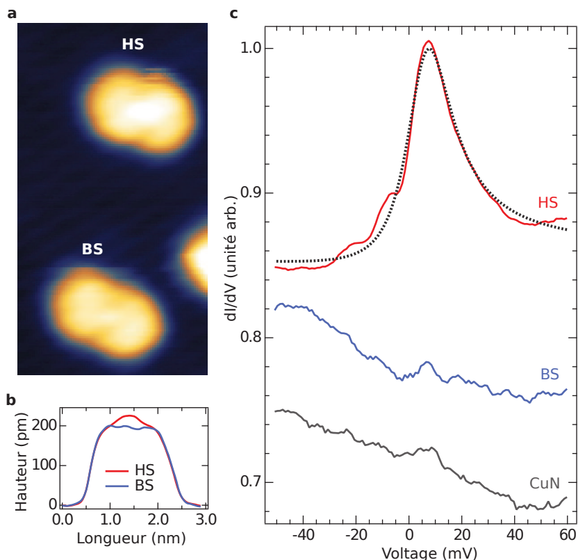
Figure XII. – Identification des états de spin des molécules de Fe-phen sur une surface de CuN/Cu(100). a, Topographie montrant deux molécules de Fe-phen dans des conformations différentes. b, Profils de hauteur permettant de mieux visualiser les deux différentes conformations. c, Spectres dI/dV mesurés sur les deux molécules présentées en a et sur le substrat de CuN/Cu(100). L'image a une taille de 3.0 nm \times 5.5 nm.
