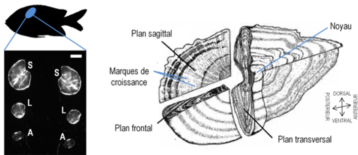
FIGURE 1.2 À gauche : Les trois paires d'otolithes d'un juvénile de Dascyllus aruanus . S : sagitta , L : lapillus , A : astericus . Barre d'échelle = 200 \mu\text{m} . À droite : Section à travers un sagitta montrant les trois plans d'orientation typiques et indiquant des marques de croissance et la localisation du noyau (modifié d'après Panfili et al. (2002) ).
