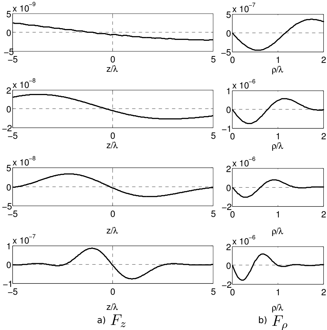
FIGURE 39 – Influence de la focalisation. Effet de l’augmentation de l’angle d’ouverture (de haut en bas \alpha_0 = 19,5^\circ, 30^\circ, 39^\circ et 56,5^\circ ) sur la force axiale F_z en (a) et radiale F_\rho en (b). Les forces sont données en newtons.
