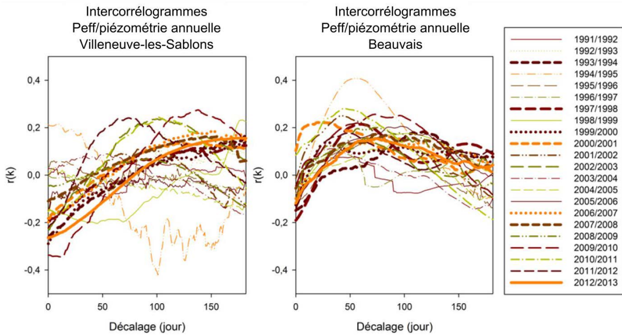
Figure 6-17 : Intercorrélogrammes Peff-piézométrie annuels à Beauvais et Villeneuve-les-sablons (1991-2013).
