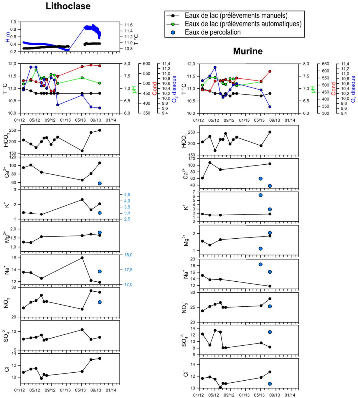
Figure 4-17 : Lac de la Lithoclase et lac Murine ; Paramètres physicochimiques des eaux des lacs (Température, pH, Conductivité électrique, et concentration en Oxygène dissous en \text{mg L}^{-1} ) ; Concentrations en ions majeurs ( \text{HCO}_3^- , \text{Ca}^{2+} , \text{K}^+ , \text{Mg}^{2+} , \text{Na}^+ , \text{NO}_3^- , \text{SO}_4^{2-} , \text{Cl}^- ) des eaux des lacs (prélèvements manuels en noir) et des eaux de percolation (en bleu) en \text{mg L}^{-1} .
