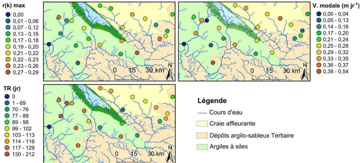
Figure 6-22 : Distribution spatiale des r(k)_{max} , des TR et des Vm des intercorrélogrammes Peff/piézométrie (période 2009/2014) pour les 22 piézomètres situés dans la craie libre du Nord-Ouest du Bassin de Paris.
