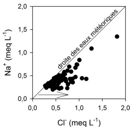
Figure 6-5 : \text{Na}^+ vs \text{Cl}^- ( \text{meq L}^{-1} ). La droite théorique des eaux météorique est représentée en noir.
