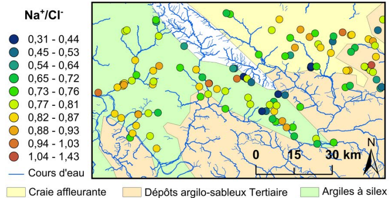
Figure 6-6 : Distribution spatiale des ratios \text{Na}^+/\text{Cl}^- et des formations superficielles.
