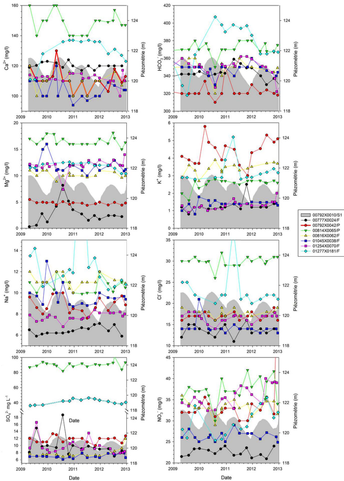
Figure 6-26 : Variations temporelles des concentrations en ions majeurs en mg L -1 de 7 qualitomètres comparées à la variation de la piézométrie de la nappe de la craie enregistrée par le piézomètre 00792X0010/S1 (données de la Banque ADES).
