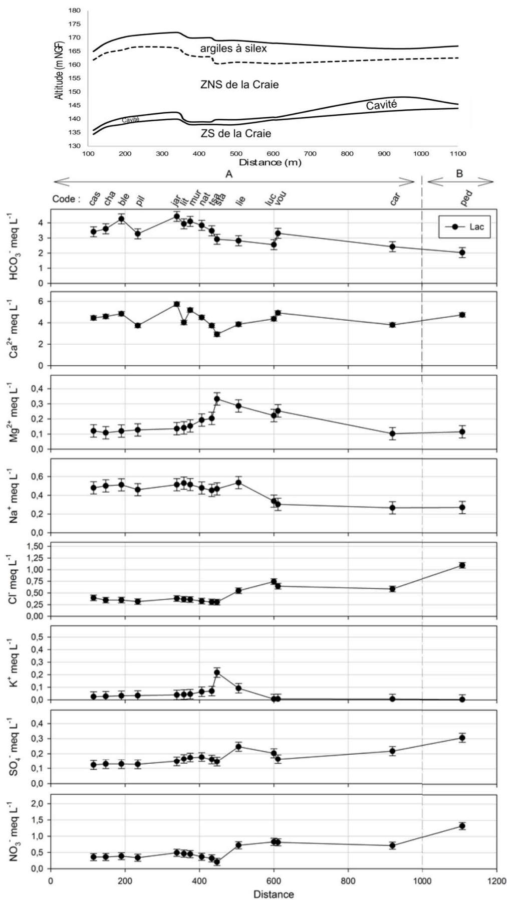
Figure 7-2 : Hétérogénéité spatiale de la concentration en ions majeurs des eaux des lacs prélevés lors d'une campagne en juillet 2013 et coupe schématique de la ZNS au-dessus de la cavité.
