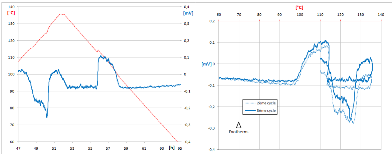
Figure 4-27 : 3 ème cycle à 6°C/h pour le même échantillon de 390 g de \text{MgCl}_2 \cdot 6\text{H}_2\text{O}
