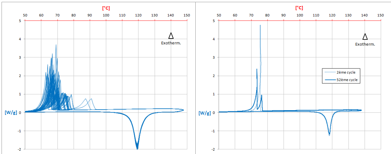
Figure 3-28 : 49 cycles à 5°C/min + 52 ème cycle à 2°C/min pour 20,4 mg de MgCl 2 .6H 2 O (C.I.D.) Note : Cet essai a été réalisé avec les coefficients d'étalonnage présentés par le Tableau 3-7 de la page 68.
