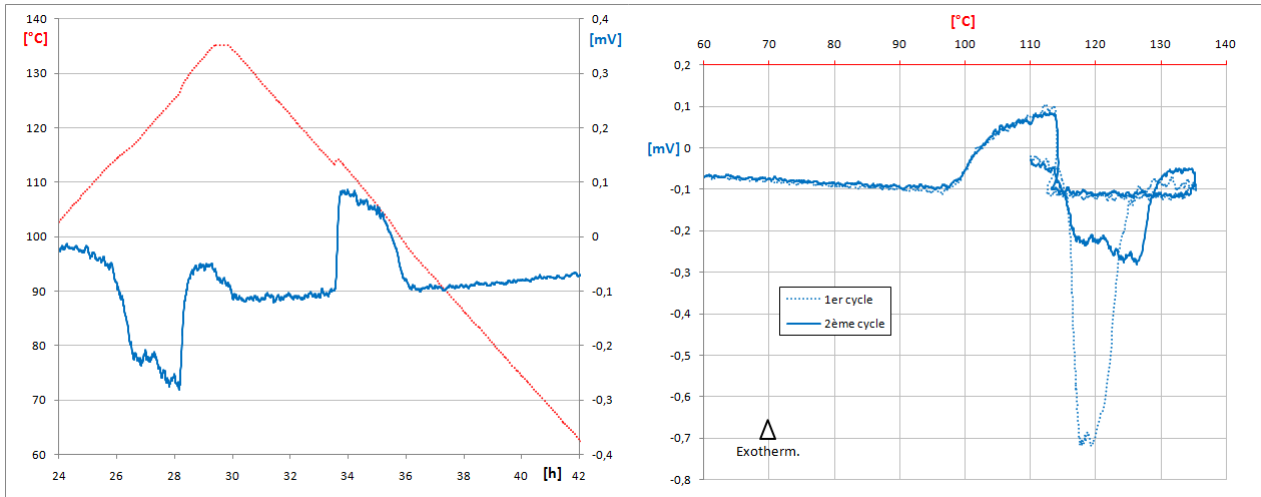
Figure 4-26 : 2 ème cycle à 6°C/h pour un échantillon de 390 g de \text{MgCl}_2 \cdot 6\text{H}_2\text{O}
