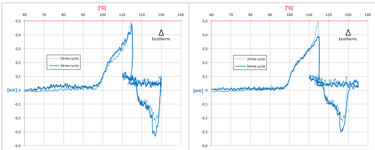
Figure 4-24 : 3 ème et 5 ème cycle à 6°C/h pour le même échantillon de 469 g de MgCl 2 .6H 2 O
