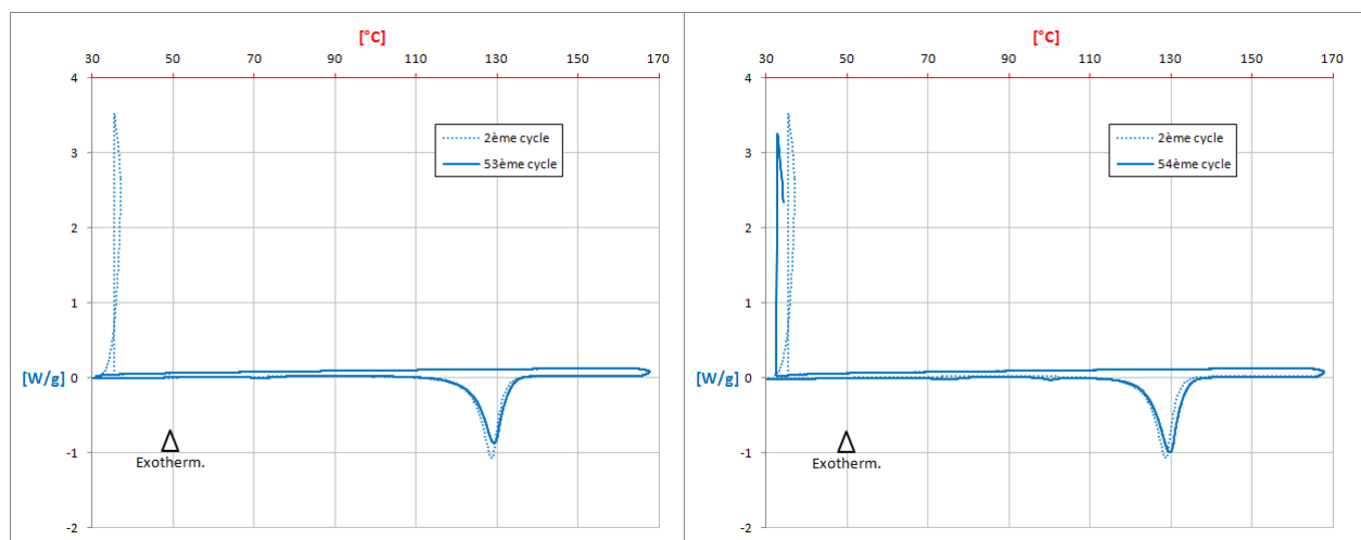
Figure 3-41 : 53 ème cycle à 2°C/min (après court repos) + 54 ème cycle à 2°C/min (après long repos)
