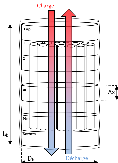
Figure 7-19 : Discretisation spatiale d'une cuve verticale remplie de nodules cylindriques
