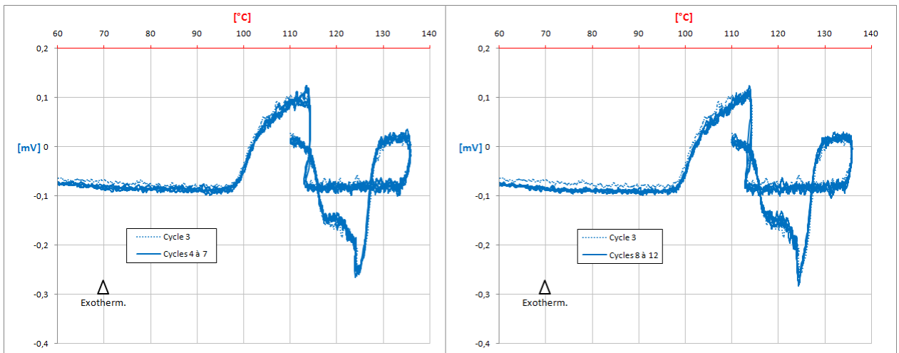
Figure 4-28 : Cycles 4 à 7 et 8 à 12, réalisés à 6°C/h pour 390 g de \text{MgCl}_2 \cdot 6\text{H}_2\text{O}
