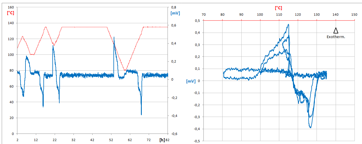
Figure 4-25 : Cycles 6 à 9, réalisés à 6°C/h pour 469 g de MgCl 2 .6H 2 O avec fusion puis cristallisation incomplète
