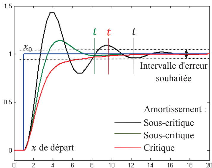
Figure 20: Oscillation des ressorts différents avec des amortissements différents.
