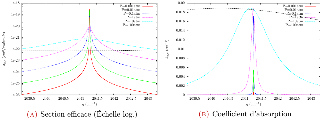
FIGURE 2.14 – Effet de la pression sur la section efficace (donnée avec une échelle logarithmique) et le coefficient d'absorption d'une raie de \text{CO}_2 isolée centrée en \eta_0 = 2041.288360\text{cm}^{-1} à une température de 300\text{K} . La fraction molaire de \text{CO}_2 est de \chi_{\text{CO}_2} = 0.1 et le profil de raie considéré est un profil de Voigt.
