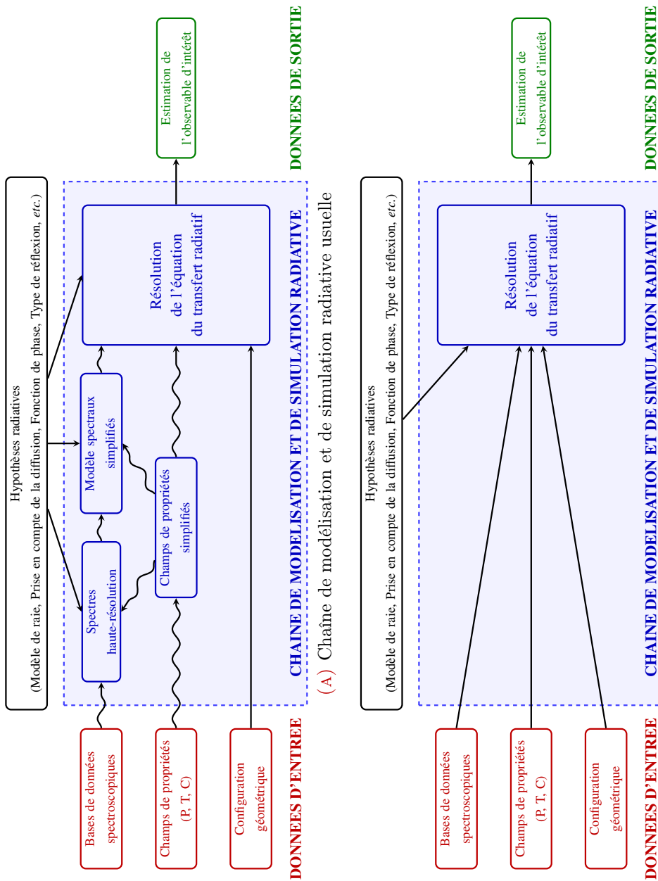
FIGURE 6.1 – Les algorithmes à collisions nulles permettent de supprimer toute approximation (symbolisées par des flèches courbes) liée à la description et la prise en compte des propriétés du milieu. Les méthodes de discrétisation (production de spectres haute-résolution, maillage volumique du milieu participant), les modèles spectraux approchés et les procédures d'interpolation, généralement employées pour évaluer localement les propriétés radiatives, sont ainsi évitées.
