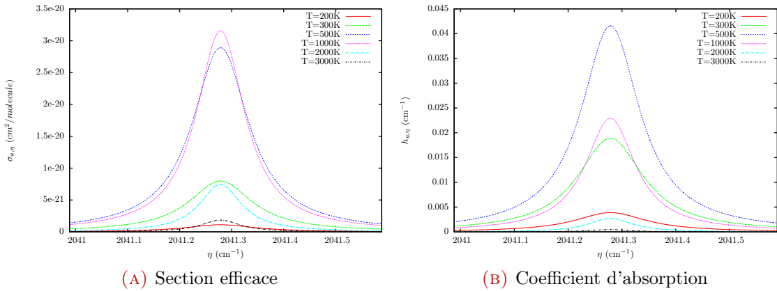
FIGURE 2.15 – Effet de la température sur la section efficace et le coefficient d'absorption d'une raie de \text{CO}_2 isolée centrée en \eta_0 = 2041.288360\text{cm}^{-1} . La fraction molaire de \text{CO}_2 est fixée à \chi_{\text{CO}_2} = 0.1 , la pression à 1\text{atm} et le profil de raie considéré est un profil de Voigt.
