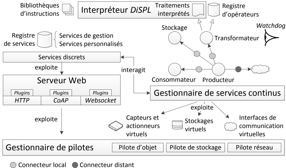
FIGURE 4.1 – Architecture de l'intergiciel Diopase .
