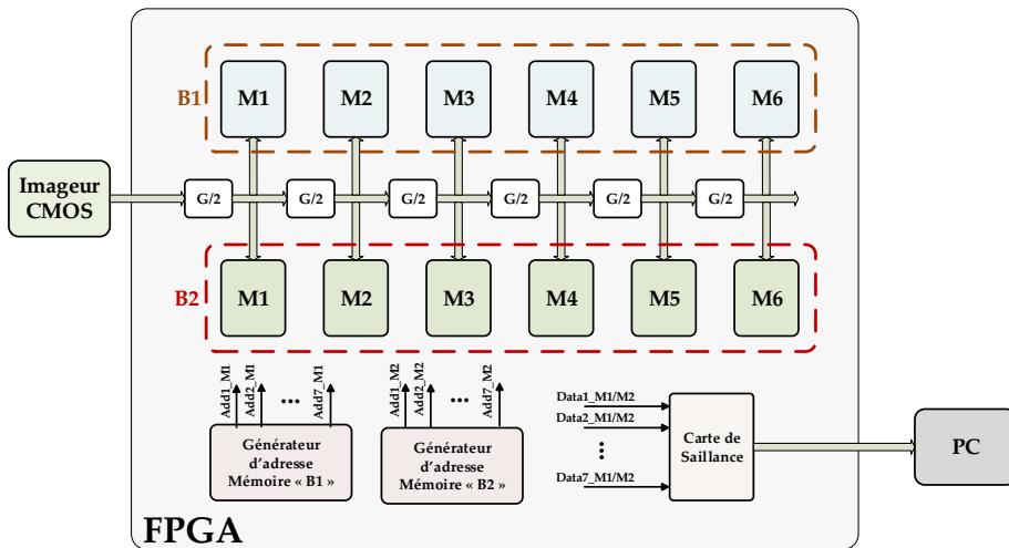
FIGURE 6.1: Architecture détection de saillance proche mémoire.
