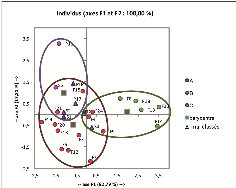
Figure 36-a : Analyse discriminante des données hydrochimiques : classification par 'lithologie'
