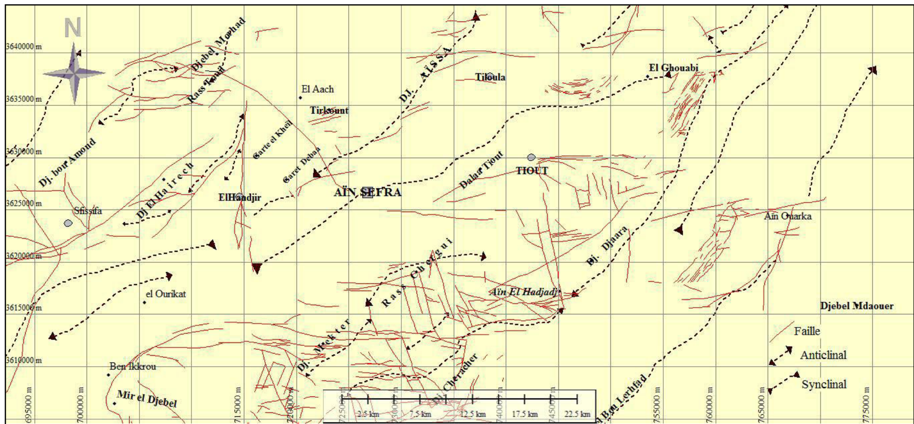
Figure 10 : Carte structurale de la partie occidentale et centrale des Monts des Ksour (base de la carte photogéologique de D. Galmier 1972, et l'accident Ras Touil-Aïn Séfra)
