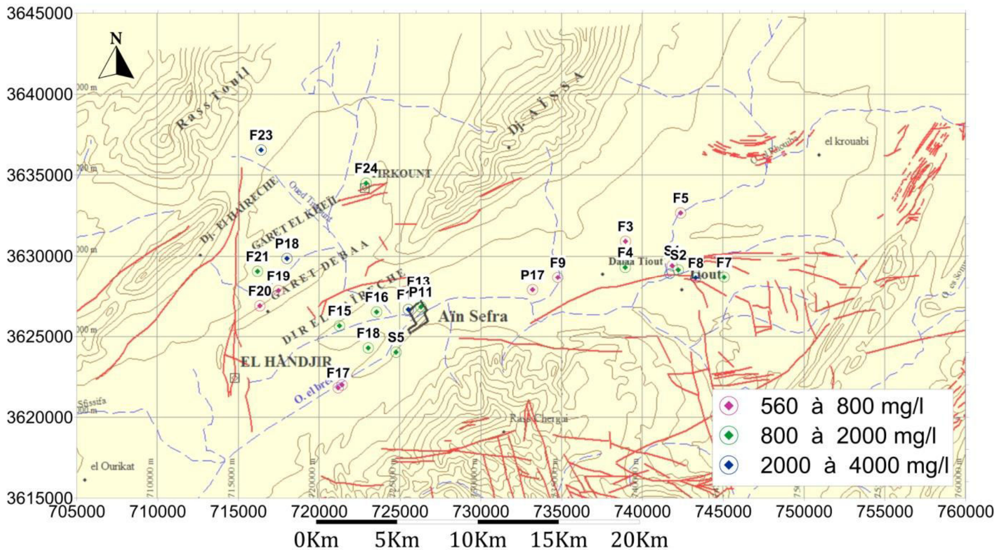
Figure 33 : Distribution de la minéralisation des eaux des gouttières synclinales d'Aïn Séfra
