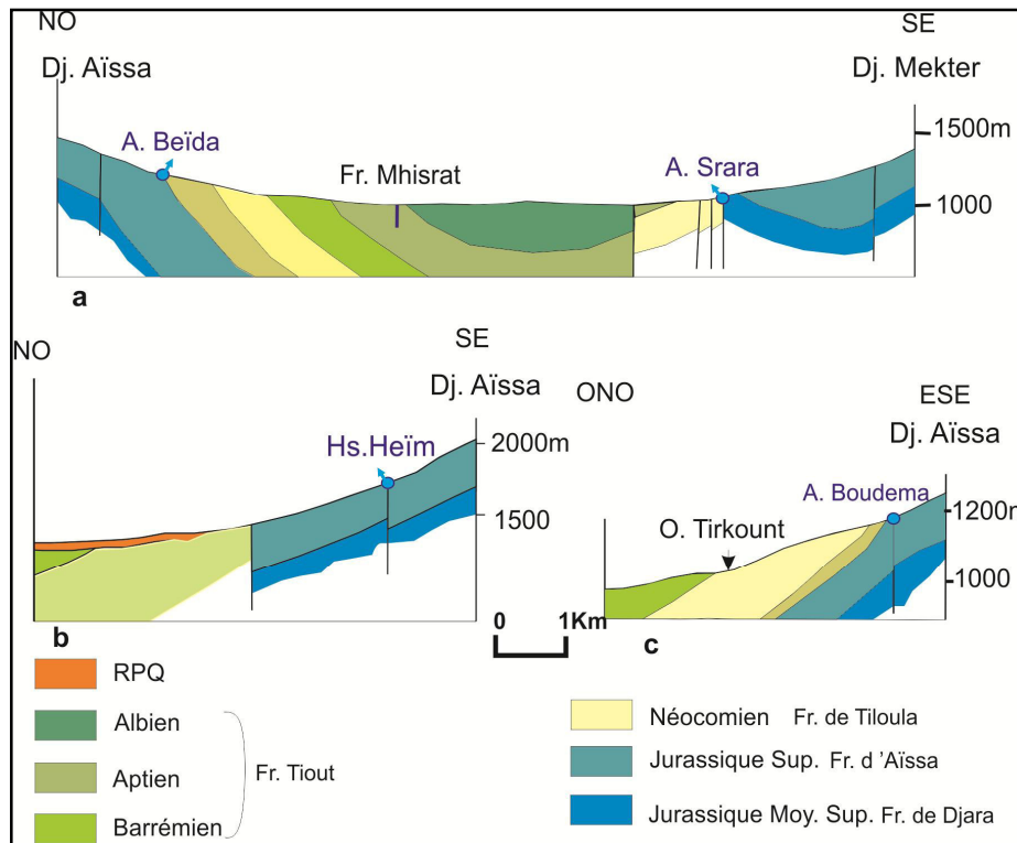
Figure 13 : Mécanismes d'émergence des sources du Jurassique a : Aïn Beïda Aïn Srara, b : Hassi Haïm, c : Aïn Boudema
