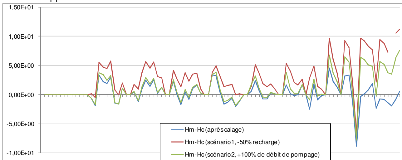
Figure 40 : Représentation des H de la simulation en régime permanent, premier et second scénarios.
