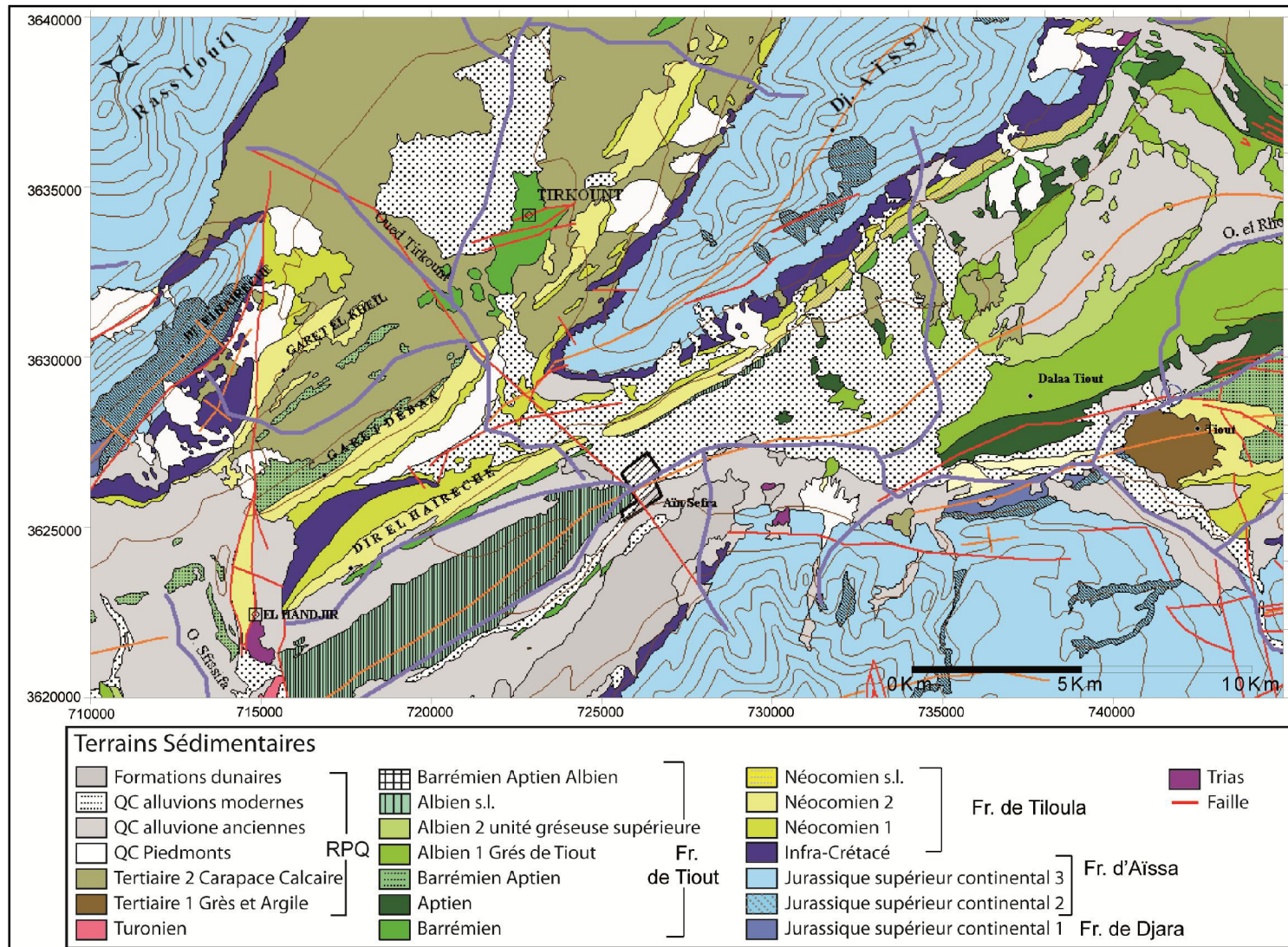
Figure 3: Carte géologique de la région d'Aïn Séfra (D. Galmier 1972)
