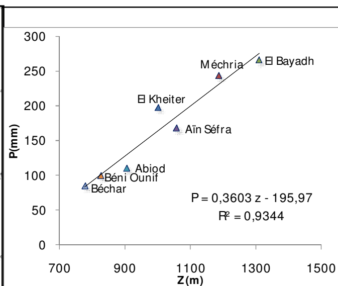
Figure 25-b : Gradient pluviométrique des Monts des Ksour
