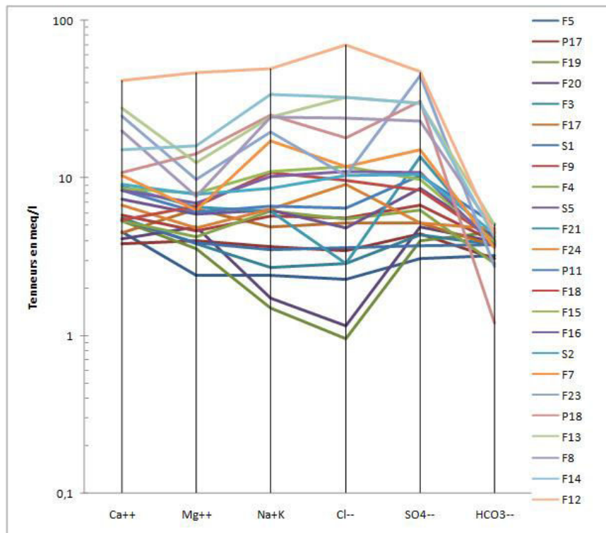
Figure 32 : Diagramme logarithmique vertical. Eaux de la région d'Aïn Séfra
