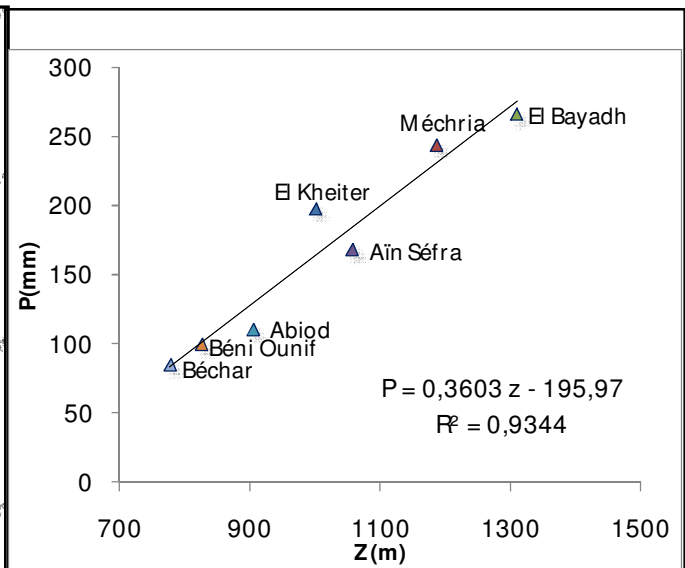
Figure 25-b : Gradient pluviométrique des Monts des Ksour
