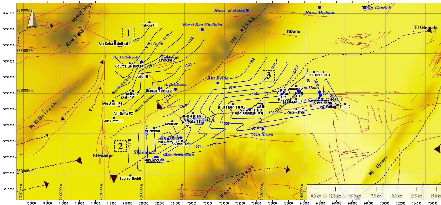
Figure 20 : Carte piézométrique du synclinale d'Aïn Séfra (septembre 2008)
