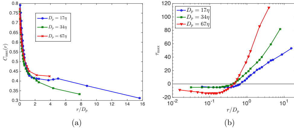
FIGURE 2.11 – (a) Valeur maximale de l'anti-corrélation entre la force et la direction de glissement, en fonction de la distance à la surface de la particule r , pour les trois diamètres de particule considérés. (b) Décalage temporel \tau_{\max} pour lequel cette anti-corrélation est maximale en fonction de la distance r .
