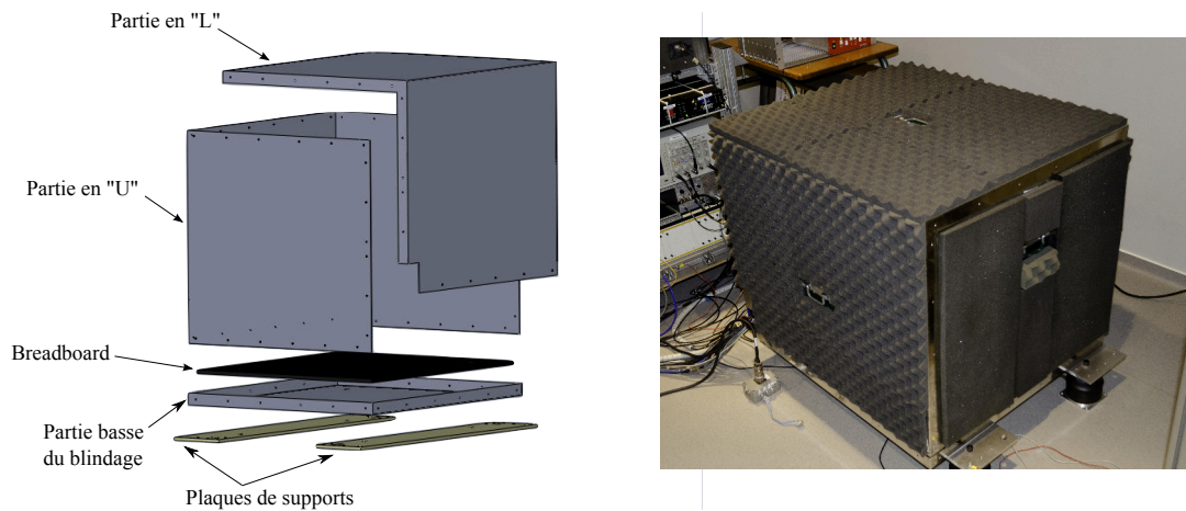
Figure 2.17 À gauche, vue en éclaté du blindage. Les plaques de support pour l'interface avec les rails de l'avion, la partie basse du blindage et le breadboard sont assemblées avec 4 vis M12 en titane. Les parties "U" et "L" du blindage peuvent être assemblées avec le reste par le biais de vis adaptées, comme le représente la photo de droite. Le blindage est recouvert de mousse afin de le protéger de tout choc éventuel.
