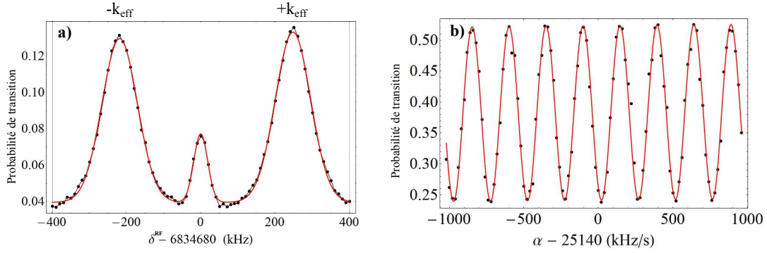
Figure 1.6 a) Spectroscopie Raman après un temps de vol d'environ 10 ms. Les deux transitions \pm k_{eff} sont bien séparés. Le pic du milieu est seulement dû à une transition Raman co-propageante résiduelle. b) Franges d'interférences obtenues sur la transition +k_{eff} en variant la rampe de fréquence \alpha .
