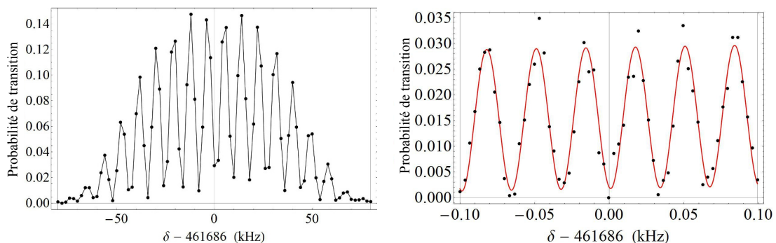
Figure 4.12 A gauche, franges de Ramsey Potassium obtenues au laboratoire sur l'axe Z avec T = 100 \mu\text{s} . À droite, franges obtenues dans les mêmes conditions avec T = 30 \text{ ms} , le contraste est plus faible suite à la chute des atomes hors de l'angle solide de détection de la photodiode.
