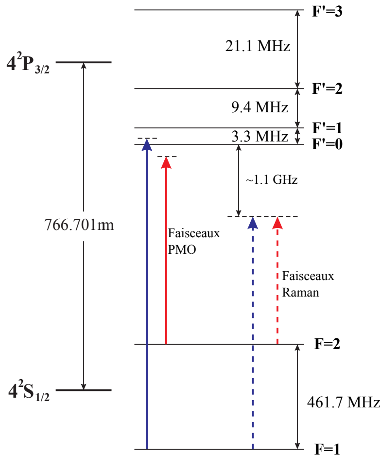
Figure 3.7 Structure atomique du Potassium 39
