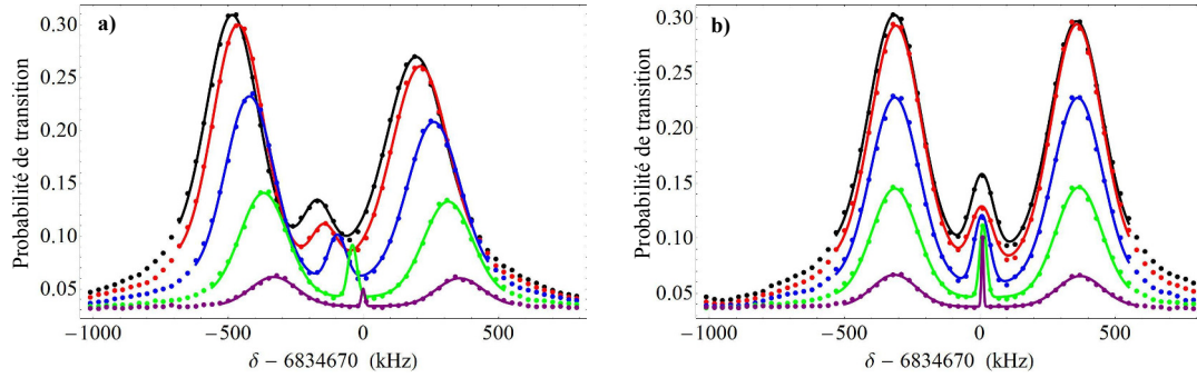
Figure 4.7 a) Spectres Raman pour différentes intensités et pour un ratio I_2/I_1 \approx 0.14 , le déplacement lumineux n'est alors pas compensé. b) Mêmes mesures que précédemment, mais avec un ratio I_2/I_1 \approx 0.62 , qui permet de compenser le déplacement lumineux. On remarque que plus la durée du pulse est grande (conservation des conditions d'un pulse \pi ), plus l'amplitude diminue, ceci est dû à la sélectivité en vitesse de la transition Raman, qui adresse une classe d'atome de plus en plus petite.
