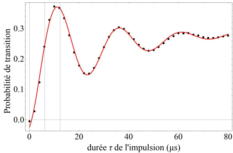
Figure 4.4 Oscillation de Rabi d'impulsion Raman contra-propageants. L'ajustement donne des pulses \pi et \pi/2 d'une durée de 12.6 \mu\text{s} et 5.8 \mu\text{s} respectivement (lignes grises verticales).
