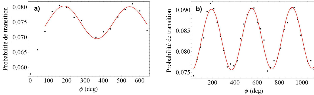
Figure 4.2 a) Franges contra-propageantes durant une parabole. L'ajustement sinusoidal est représenté en rouge, seulement pour les points acquis en 0g, et donne un SNR \approx 9 . b) Franges contra-propageantes acquises au sol dans l'avion, la semaine précédant les vols. L'ajustement donne un SNR \approx 14 .
