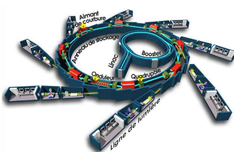
Figure 1 : représentation schématique des divers composants du synchrotron SOLEIL (Source : www.synchrotron-soleil.fr/images/File/RessourcesPedagogiques )
