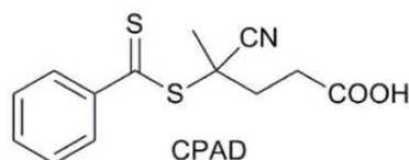
Figure 10 : Agent de transfert RAFT porteur d'une fonction acide carboxylique : le 4-Cyano-4-(phénylcarbonothioylthio)pentanoic acid (CPAD)
