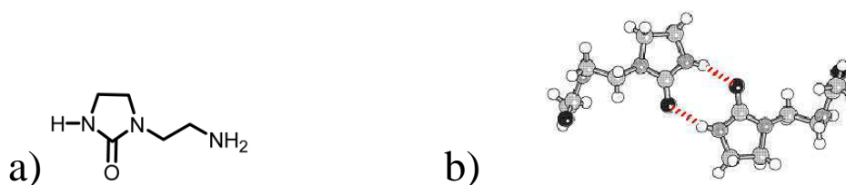
Figure 1 : (a) Représentation chimique de la molécule d'UDETA (b) Représentation de la liaison hydrogène entre deux fonctions imidazolidones obtenue à partir de la structure cristalline connue d'un dérivé de UDETA (noir : N, blanc : H, gris : C).
