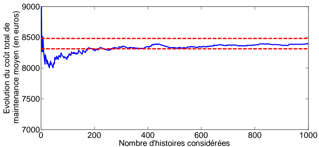
Figure 4.8: Illustration de la convergence de l'estimation du C_{TM} en fonction du nombre d'histoires (MFOP=50000 km et un NC=90\% )
