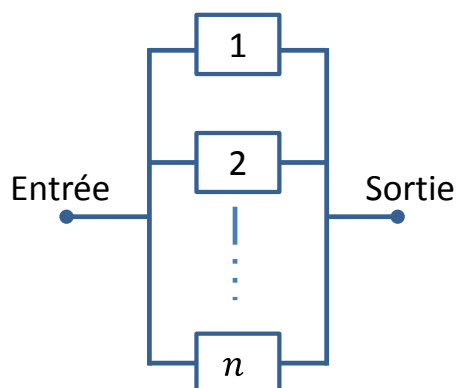
Figure 2.12: Diagramme de fiabilité d'un système parallèle
