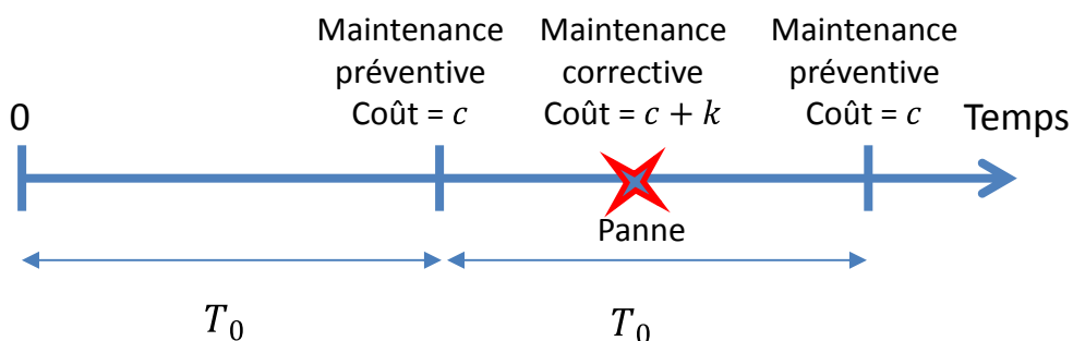
Figure 3.6: Schéma d'une politique de remplacement par bloc
