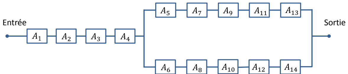
Figure 5.7: Structure du système multi-composant
