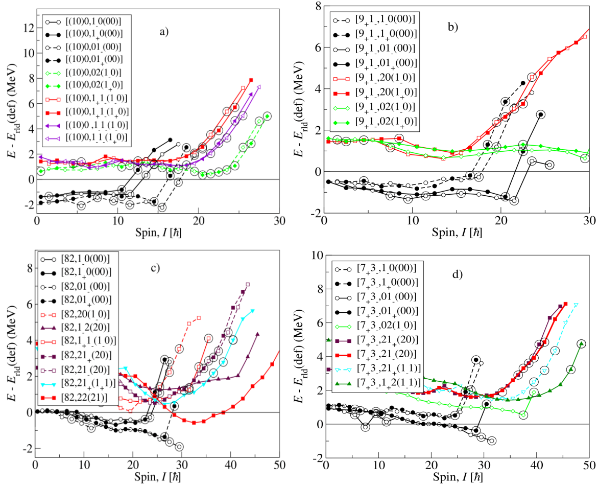
Figure 5.7 : Énergies relatives à une goutte liquide en rotation calculées pour les configurations suivantes : a) [(10)0, (n_1)_{\alpha_1} (n_2)_{\alpha_2} ((n_3)_{\alpha_3} (n_4)_{\alpha_4})] , i.e. les configurations avec 10 protons de valence dans l'orbitale ( dg ), b) [9_+1_1, (n_1)_{\alpha_1} (n_2)_{\alpha_2} ((n_3)_{\alpha_3} (n_4)_{\alpha_4})] , c) [82, (n_1)_{\alpha_1} (n_2)_{\alpha_2} ((n_3)_{\alpha_3} (n_4)_{\alpha_4})] , d) [7_+3_-, (n_1)_{\alpha_1} (n_2)_{\alpha_2} ((n_3)_{\alpha_3} (n_4)_{\alpha_4})] . Avec un nombre impair de trous neutron en \frac{h_{11}}{2} , deux bandes dégénérées avec signature différente sont calculées pour chaque configuration et sont tracées en utilisant la même couleur et les mêmes symboles (pleins et ouverts).
