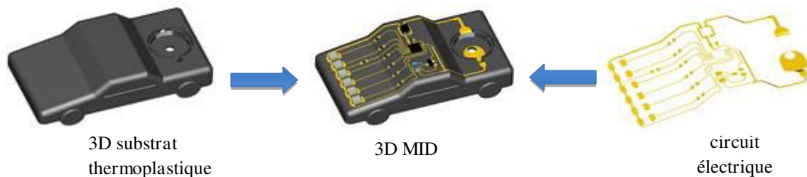
Fig. 2.1 : Principe de la technologie MID 1 .
