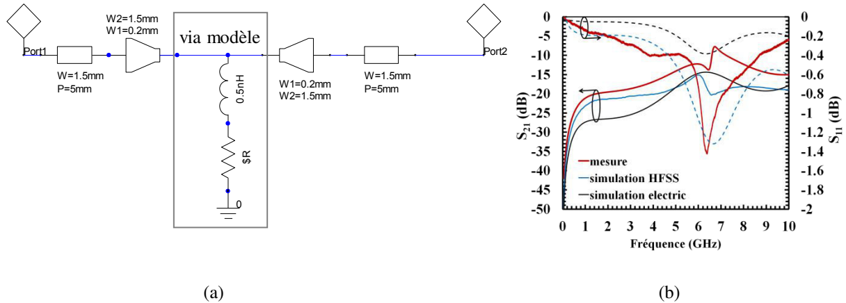
Fig. 4.5 : (a) Modèle électrique de LDS microruban via and (b) sa réponse en fréquence du S_{21} et S_{11} .
