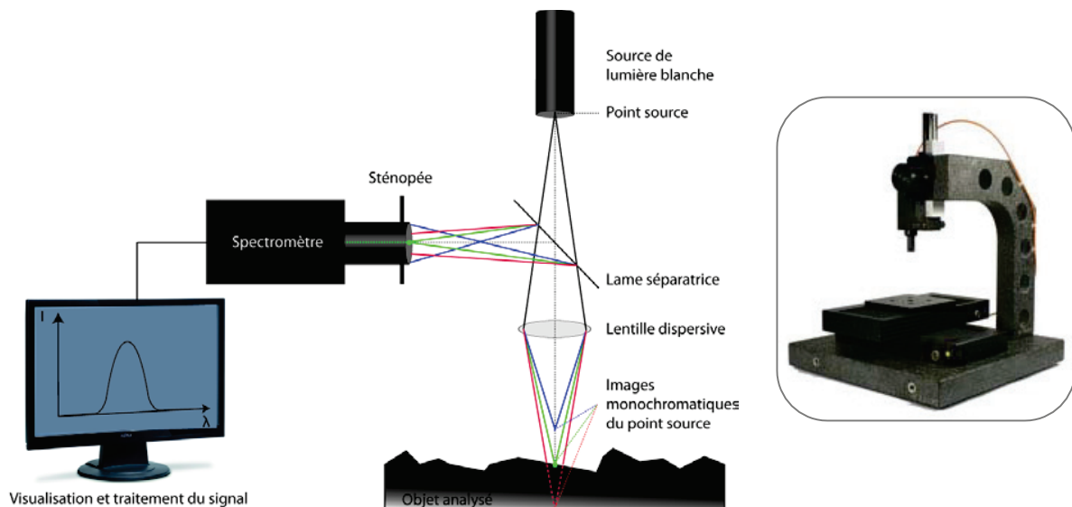
Figure 4-13. Profilomètre NJ-Optimal
