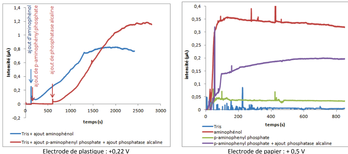
Figure 6-8. Courbes de chronoampérométrie en présence du substrat ou produit de la phosphatase alcaline Les courbes de gauche représentent l'intensité mesurée en fonction du temps, en présence de tampon tris puis d'aminophénol ou de p-aminophényl phosphate et de phosphatase alcaline, sur l'électrode de plastique avec un potentiel appliqué de +0,22 V. Celles de droites sont basées sur les mesures effectuées sur l'électrode de papier à un potentiel de +0,5 V, en présence de tampon, d'aminophénol, de p-aminophényl phosphate ou de p-aminophényl phosphate et de phosphatase alcaline.
