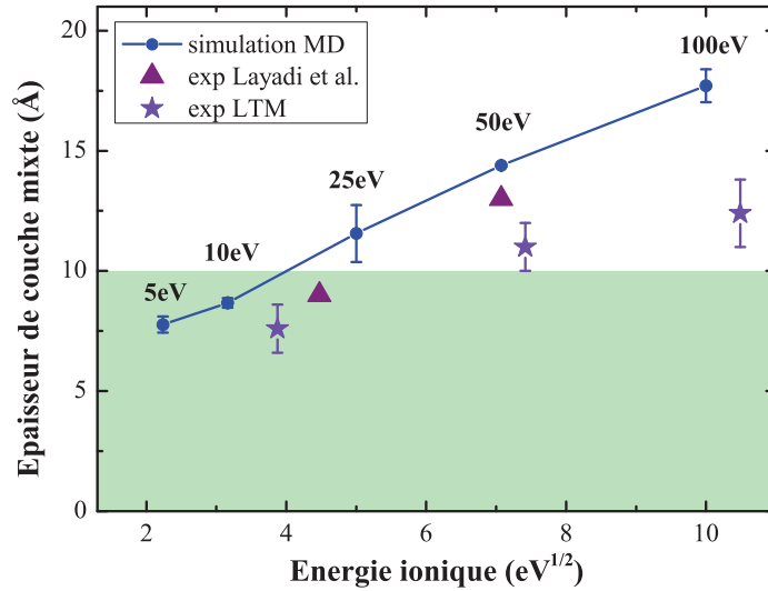
FIGURE 5.2 – Épaisseur de la couche mixte SiCl_x en fonction de l'énergie ionique à l'état stationnaire. La courbe bleue correspond aux résultats des simulations MD S_1 à S_5 (bombardement Cl/Cl^+ avec \Gamma = 100 ). Les triangles bordeaux et les étoiles violettes sont les valeurs obtenues expérimentalement par Layadi et al. [Layadi 97a, Layadi 97b] et au sein du réacteur du LTM (600 W s , 5 mTorr) [Mourey 16] (resp.) par AR-XPS et ellipsométrie.
