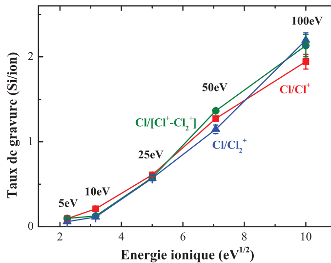
FIGURE 5.13 – Taux de gravure en fonction de l'énergie ionique pour différents types de bombardement Cl/Cl_x^+ avec \Gamma = 100 . Les neutres incidents sont toujours des radicaux Cl, seule la nature des ions ( Cl^+ ou Cl_2^+ ) varie.
