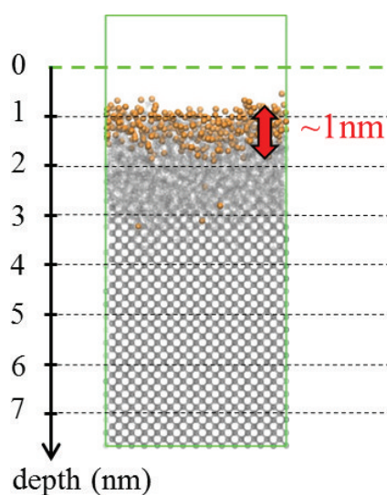
FIGURE 7.15 – Instantané de la cellule issue de l'étape 1 du cycle II, après un bombardement Cl/Cl + et pour une fluence de 0,6 \cdot 10^{15} ions/cm 2 (soit 190 ms de temps de plasma pour j = 0,5 mA/cm 2 ). La couche mixte a une épaisseur de 1 nm et contient 234 atomes de chlore.
