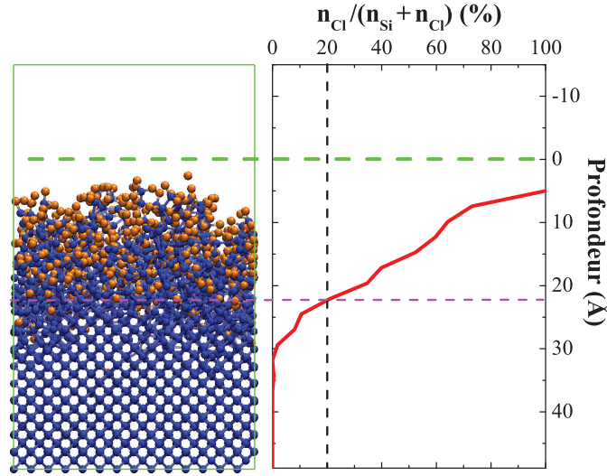
FIGURE 2.9 – Rapport des densités \frac{n_{Cl}}{n_{Si} + n_{Cl}} en fonction de la profondeur. On estime que l'interface entre la couche mixte réactive \text{SiCl}_x et le silicium bulk se situe à la profondeur en-dessous de laquelle \frac{n_{Cl}}{n_{Si} + n_{Cl}} \leq 20\% (la couche mixte contient au moins 20% de Cl).
