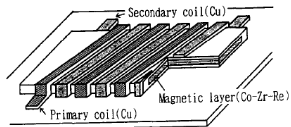
Fig.74 : Transformateur proposé par Masato.M [MYTY92]
