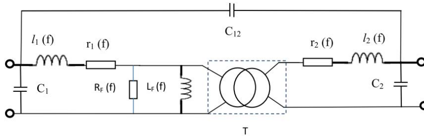
Fig.132 : Modèle haute fréquence
