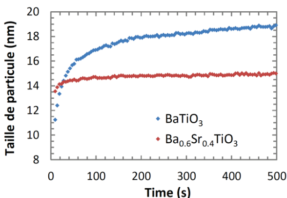
Figure 5 Etude in situ de l'influence de la substitution du baryum avec du strontium sur la croissance des particules.
