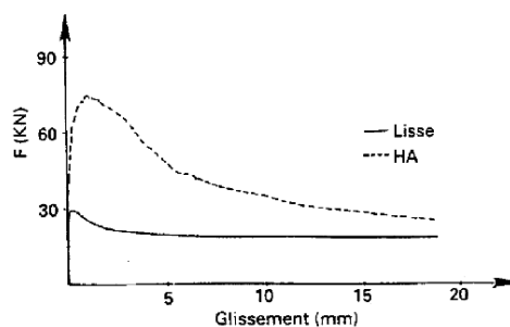
Figure 81 – Forme de la loi d'adh rence en fonction de la surface de l'armature (Hamouine et al., 1995).
