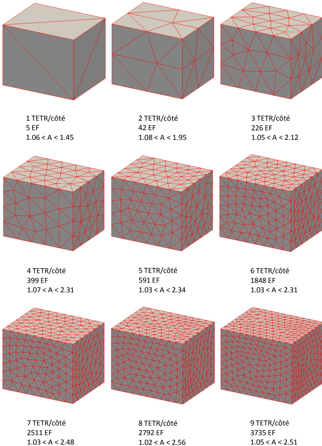
Figure 48 – Maillages du volume réalisés avec NETGEN.
