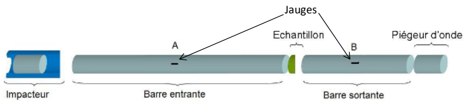
Figure 13 - Principe de l'essai de compression aux barres de Hopkinson (Safa, 2008)
