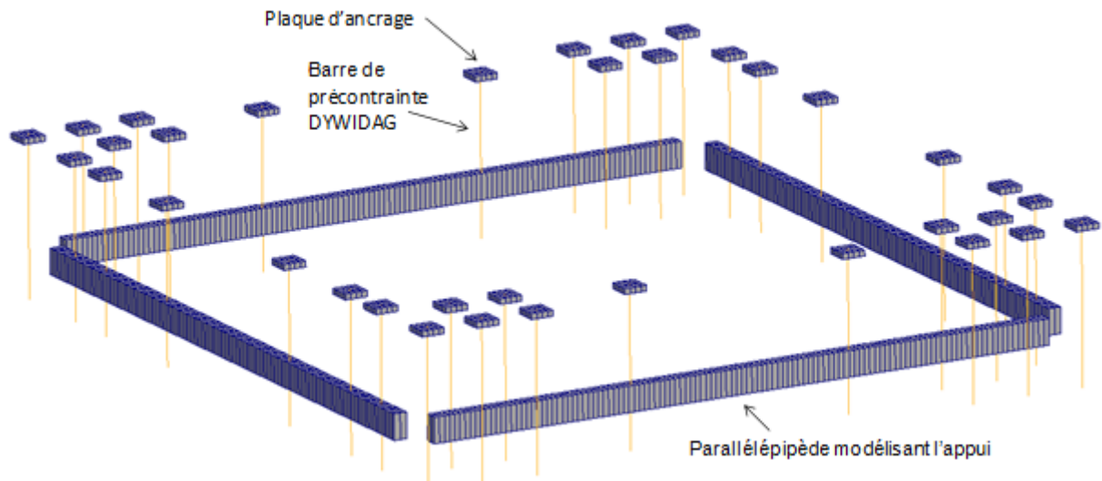
Figure 190 – Vue du maillage des appuis, des barres de précontrainte et de leurs plaques d'ancrage.
