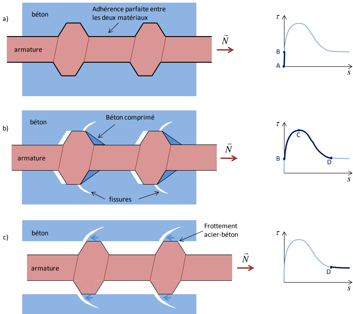
Figure 80 – D gradation de l'interface pour une armature HA (Torre-Casanova, 2012).
