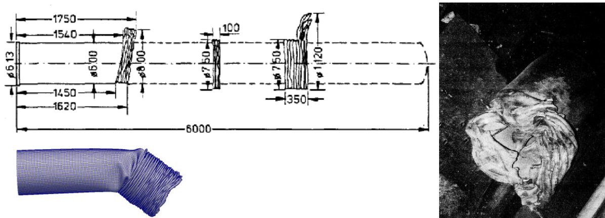
Figure 200 – Déformée du missile à la fin du calcul (en bas à gauche) et à la fin de l'essai (en haut à gauche, et à droite).
