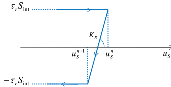
Figure 132 – Zoom sur la transition charge/décharge dans la phase 4 de la Figure 126.
