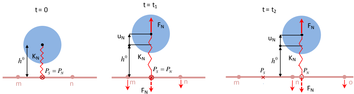
Figure 141 – Equilibre de la composante normale dans le cas d'un glissement important.
