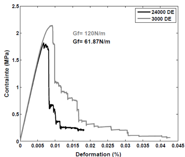
Figure 64 - Courbes contrainte-déformation lors d'un essai de traction simple pour différentes finesses du maillage ED.
