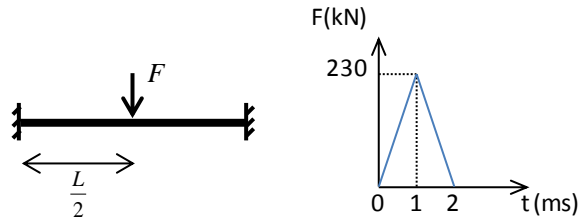
Figure 110 – Poutre en flexion encastrée à ses extrémités (à gauche) et chargement appliqué (à droite.).
