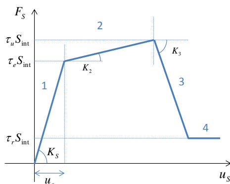
Figure 126 – Loi de comportement du lien tangentiel de la liaison acier-béton proposée par Rousseau.
