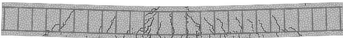
Figure 24 - Simulation d'une poutre en béton armé soumise à un impact (Kim et al., 2013).
