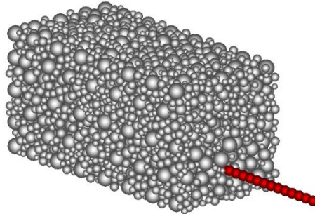
Figure 43 – Maillage éléments discrets final d'un volume de béton armé.
