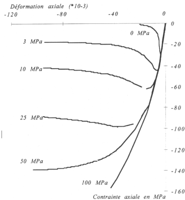
Figure 11 - Comportement triaxial du béton pour différentes pression de confinement (Jamet et al., 1984).
