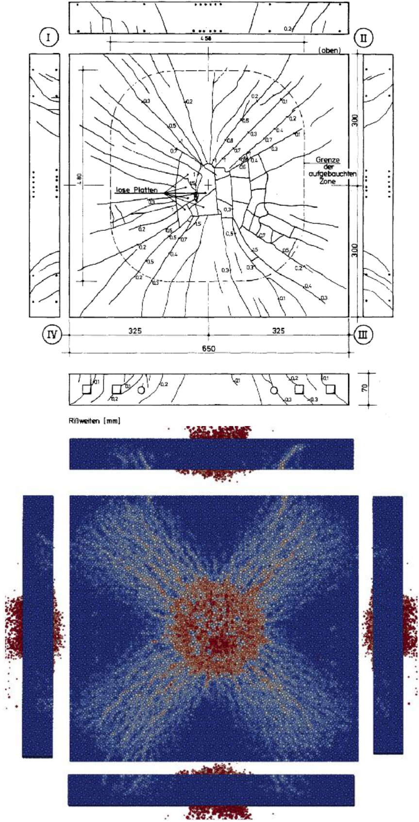
Figure 197 – Etat de fissuration final de la face arrière et des faces latérales de la dalle dans l'essai et dans le calcul.
