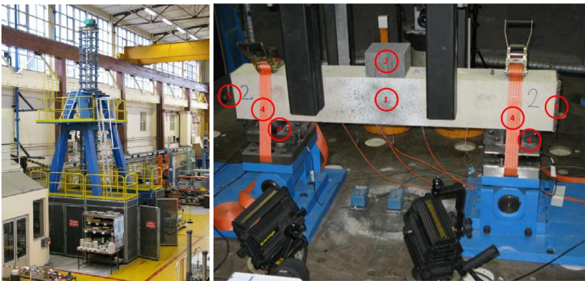
Figure 160 – Tour de chute ORION (à gauche), poutre en béton armé en position pour l'essai d'impact (à droite), (Piteau et Valin, 2011).
