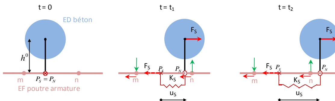
Figure 140 – Equilibre de la composante tangentielle dans le cas d'un glissement important.
