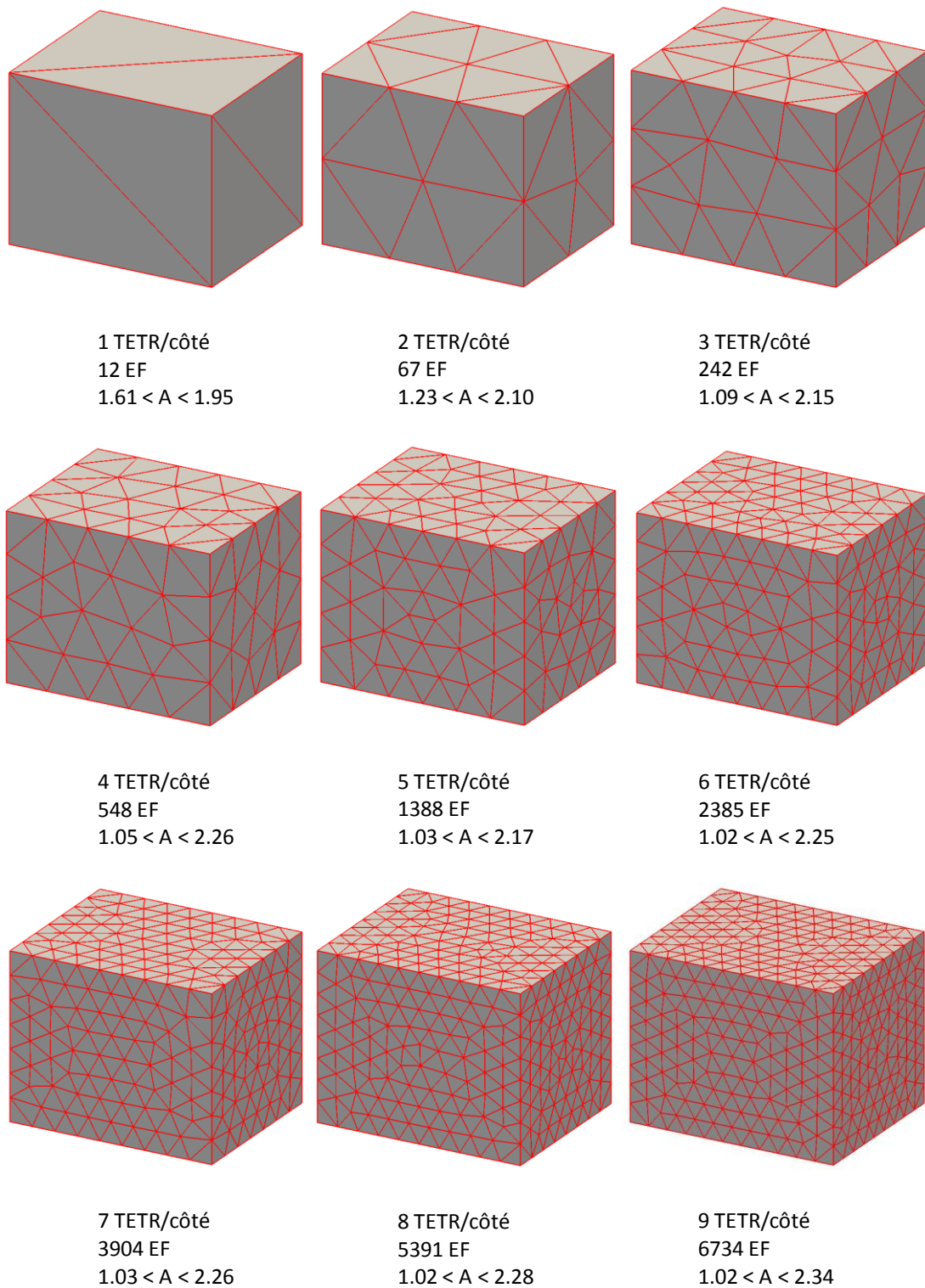
Figure 49 – Maillages du volume réalisés avec GHS3D+BLSURF.
