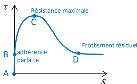
Figure 79 – Courbe typique contrainte-glisement d'un essai d'arrachement.
