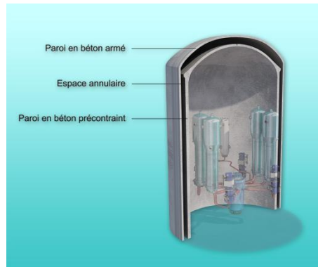
Figure 16 - Schéma d'une coupe du bâtiment réacteur (ASN).
