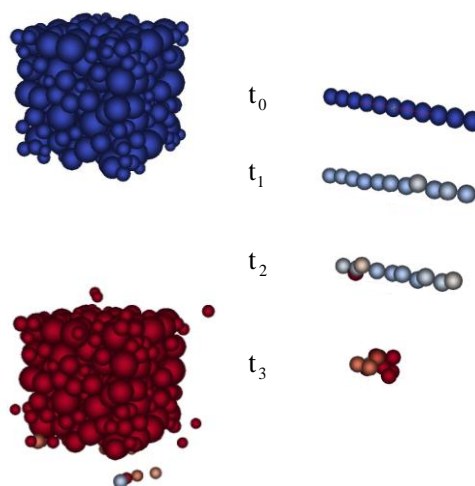
Figure 99 – États du béton et de l'armature à des instants successifs du calcul.
