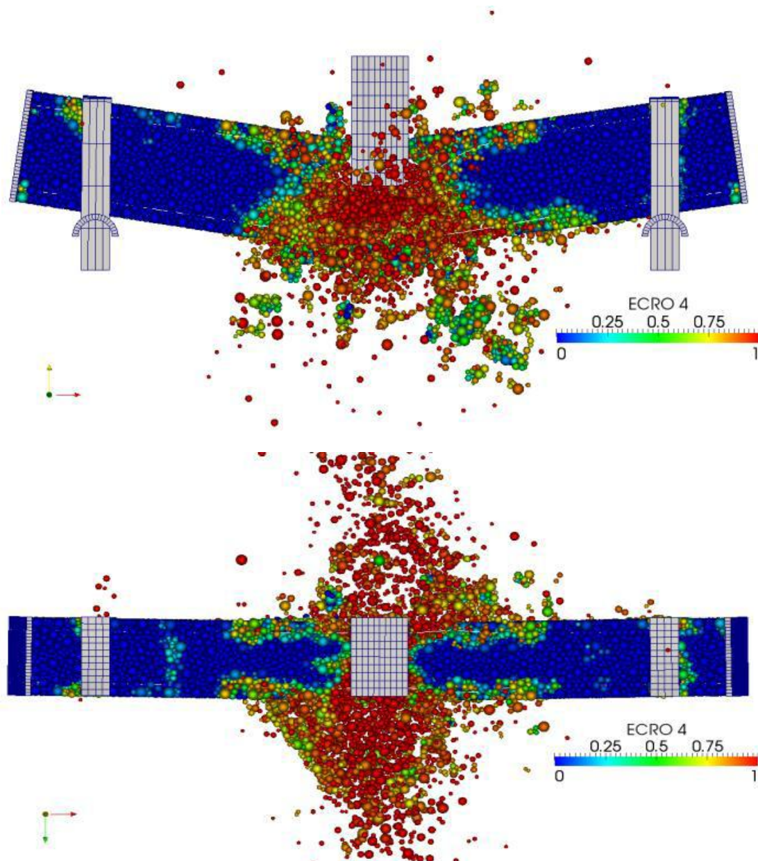
Figure 202 – Endommagement du modèle ED-EF dans le calcul sans prise en compte de l'effet de vitesse, vue de front (en haut) et de dessus (en bas).
