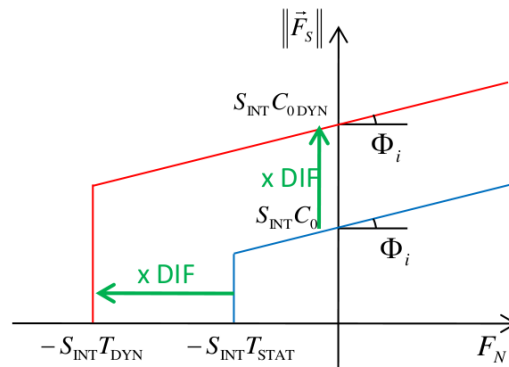
Figure 194 – Schéma du modèle de Mohr-Coulomb modifié par la loi à effet de vitesse.
