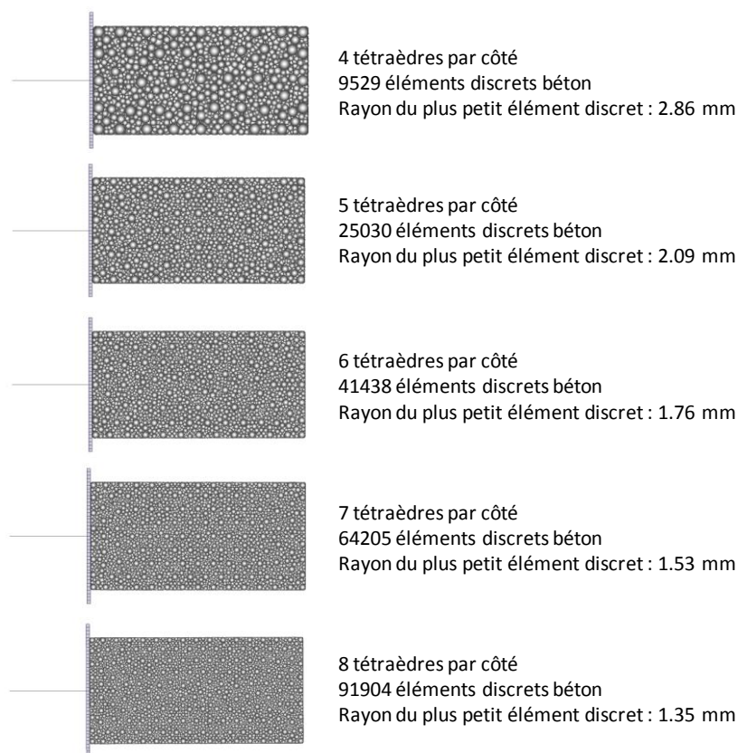
Figure 146 – Maillages ED de l'éprouvette et leurs caractéristiques.
