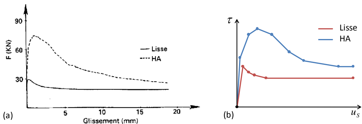
Figure 136 – (a) Courbe expérimentale (Hamouine et al., 1995) et (b) loi multipoints proposée.
