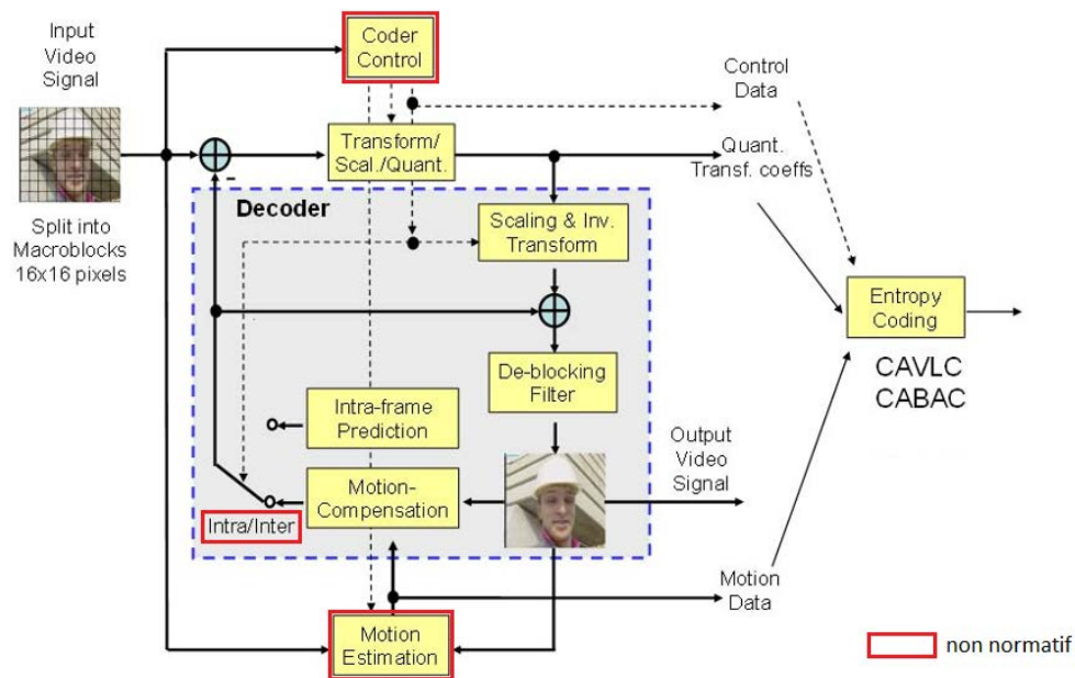
FIGURE 1.6 – Schéma d'un encodeur vidéo H.264.
