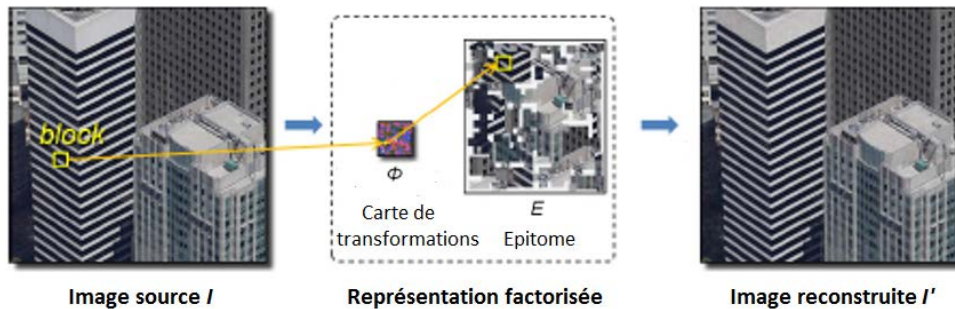
FIGURE 2.8 – Factorisation d'une image en un épitome condensé et une carte de transformations.
