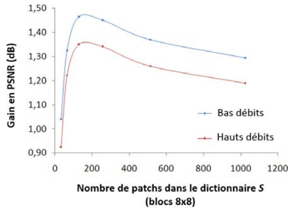
FIGURE 4.11 – Gains en PSNR par rapport à H.264 Intra versus le nombre de patches défini dans le dictionnaire S avec une taille de fenêtre de recherche fixe, pour l'image Barbara, lorsque la méthode de prédiction hybride NE/oMANE est utilisée (avec la LLE).
