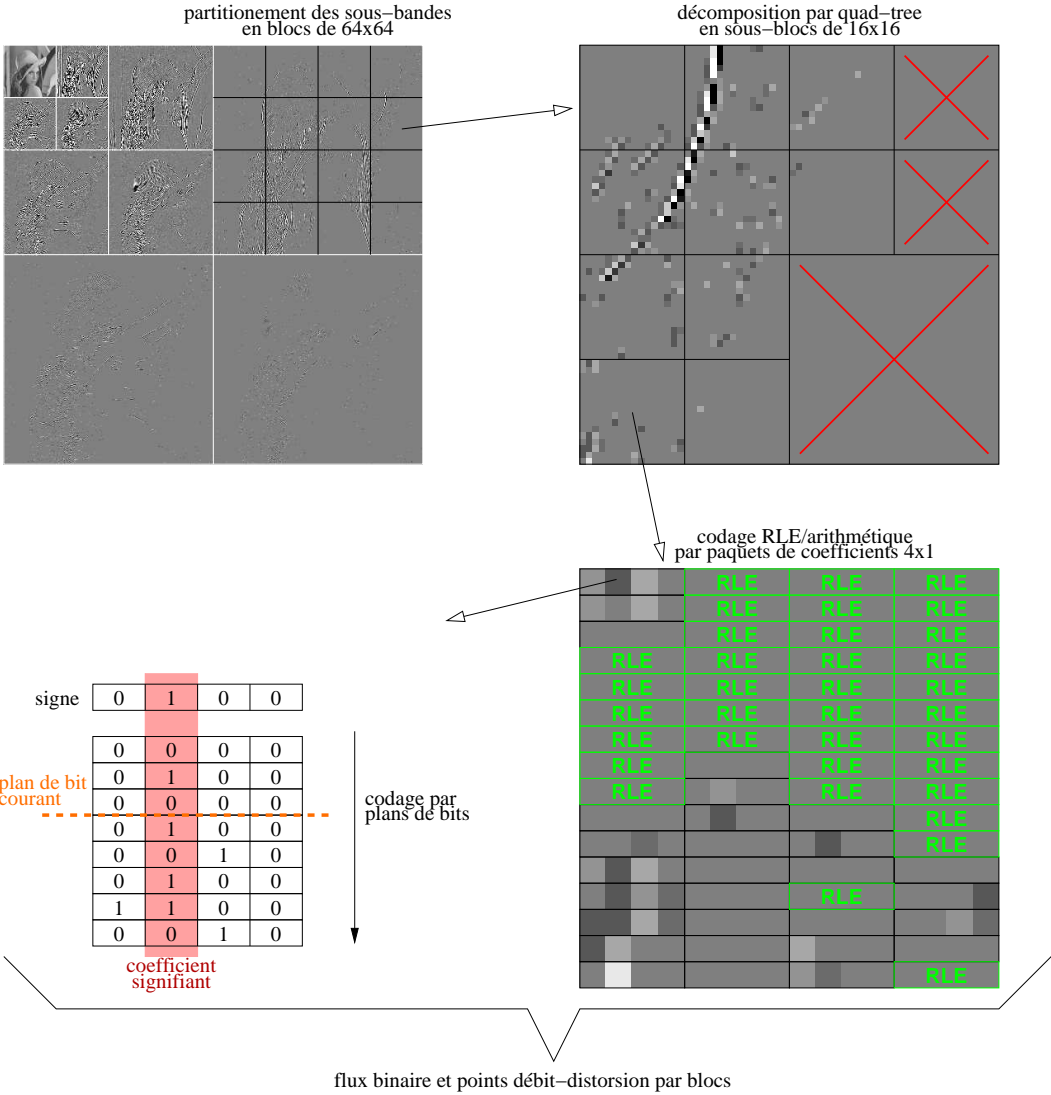
FIG. 2.7: Codage des sous-bandes d'ondelettes séparables par EBCOT. Chaque sous-bande est traitée indépendamment en la séparant tout d'abord en blocs de taille 64x64. Un quad-tree de significiance élimine rapidement les sous-blocs 16x16 insignifiants de chaque blocs. Les sous-blocs significatif sont ensuite codés par plans de bits à l'aide de deux primitives. Cette passe de codage fournit un flux binaire encodé et les valeurs de distorsion pour chaque débit.
